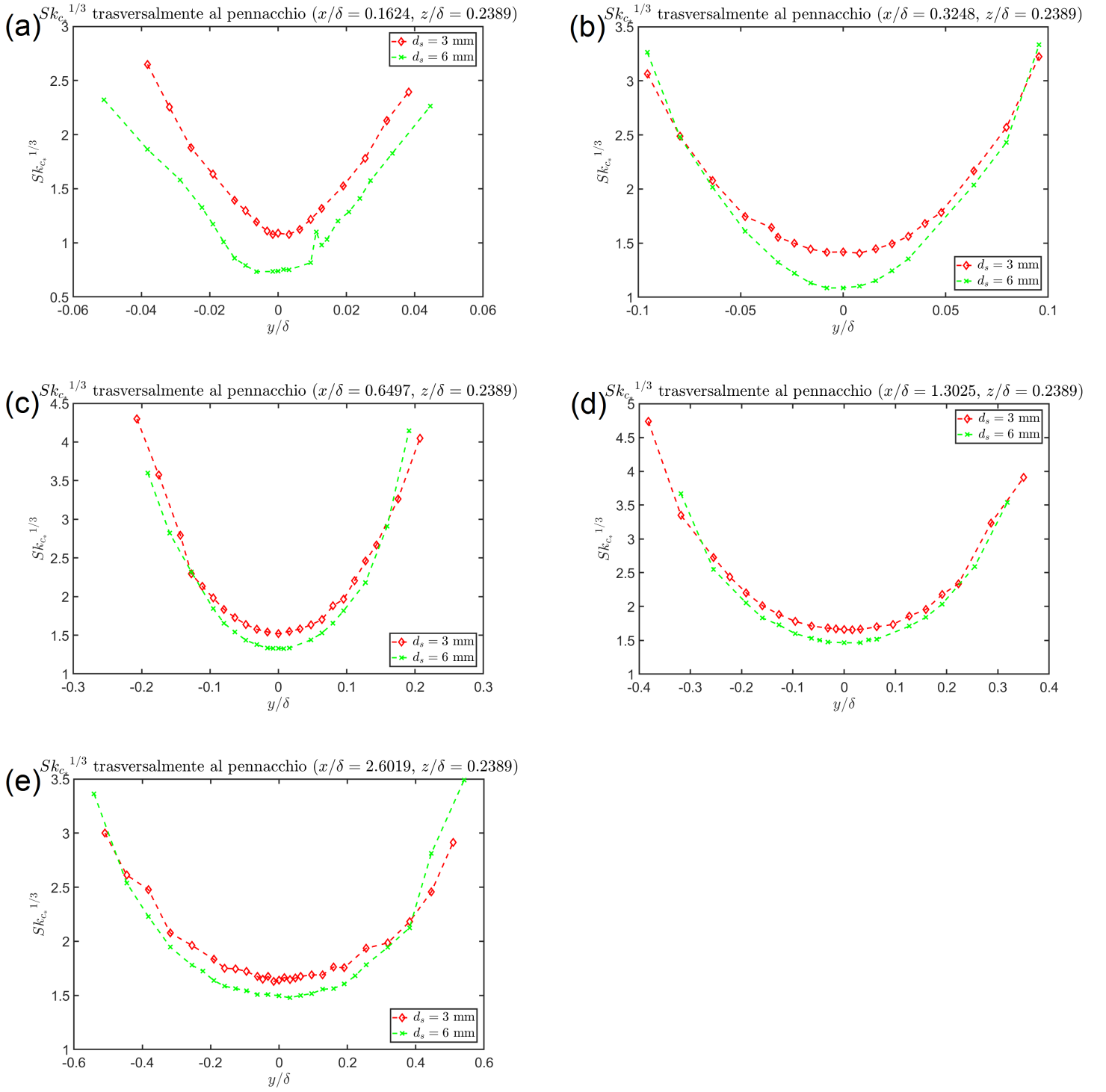
Figura 30: Grafici andamento Sk_{c*} trasversalmente al pennacchio per le cinque diverse sezioni per d_s = 3 \text{ mm} e d_s = 6 \text{ mm} , con z/\delta = 0.2389 ( z/z_s = 1 ). In particolare: (a) Andamento di Sk_{c*} per x/\delta = 0.1624 , (b) Andamento di Sk_{c*} per x/\delta = 0.3248 , (c) Andamento di Sk_{c*} per x/\delta = 0.6497 , (d) Andamento di Sk_{c*} per x/\delta = 1.3025 , (e) Andamento di Sk_{c*} per x/\delta = 2.6019
