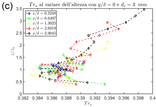
Figura 42: Grafici andamento Tr_u trasversalmente al pennacchio e al variare dell'altezza per d_s = 3 \text{ mm} e d_s = 6 \text{ mm} . In particolare: (a) Andamento di Tr_u per z/\delta = 0.2389 e d_s = 3 \text{ mm} , (b) Andamento di Tr_u per z/\delta = 0.2389 e d_s = 6 \text{ mm} , (c) Andamento di Tr_u per y/\delta = 0 e d_s = 3 \text{ mm} , (d) Andamento di Tr_u per y/\delta = 0 e d_s = 6 \text{ mm}
