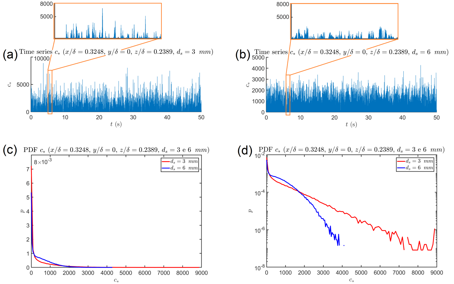
Figura 12: Grafici serie temporali e probability density functions c_* per il punto (x/\delta = 0.3248, y/\delta = 0, z/\delta = 0.2389) con d_s = 3 \text{ mm} e con d_s = 6 \text{ mm} . In particolare: (a) Serie temporale per d_s = 3 \text{ mm} , (b) Serie temporale per d_s = 6 \text{ mm} , (c) Pdf per d_s = 3 \text{ mm} e per d_s = 6 \text{ mm} , (d) Rappresentazione in scala semi-logaritmica delle pdf per d_s = 3 \text{ mm} e per d_s = 6 \text{ mm}
