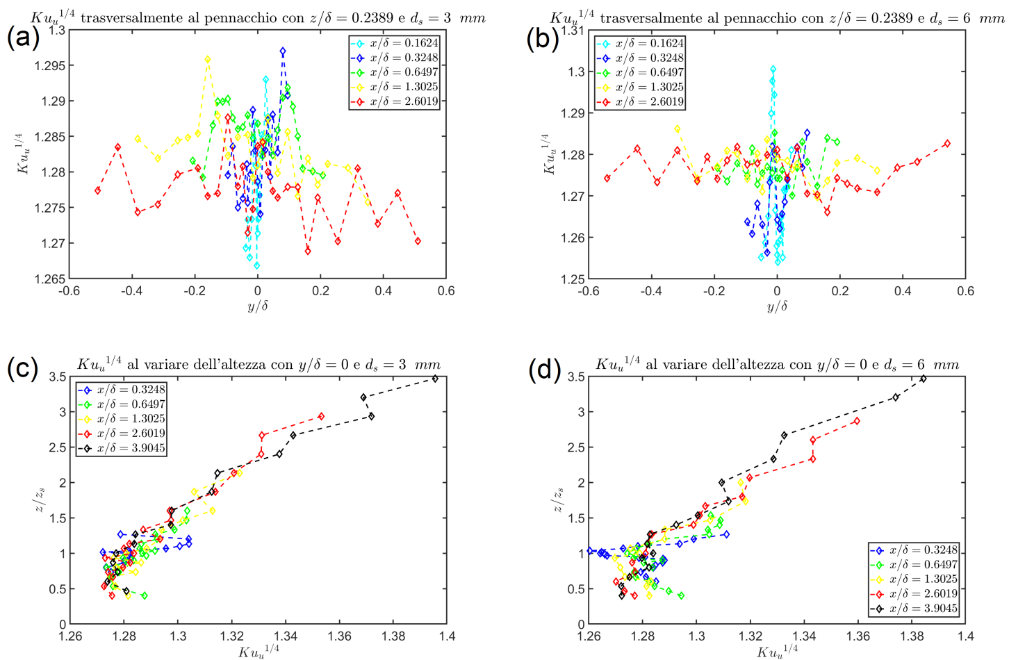
Figura 72: Grafici andamento Ku_u^{1/4} trasversalmente al pennacchio e al variare dell'altezza per d_s = 3 \text{ mm} e d_s = 6 \text{ mm} . In particolare: (a) Andamento di Ku_u^{1/4} per z/\delta = 0.2389 e d_s = 3 \text{ mm} , (b) Andamento di Ku_u^{1/4} per z/\delta = 0.2389 e d_s = 6 \text{ mm} , (c) Andamento di Ku_u^{1/4} per y/\delta = 0 e d_s = 3 \text{ mm} , (d) Andamento di Ku_u^{1/4} per y/\delta = 0 e d_s = 6 \text{ mm}
