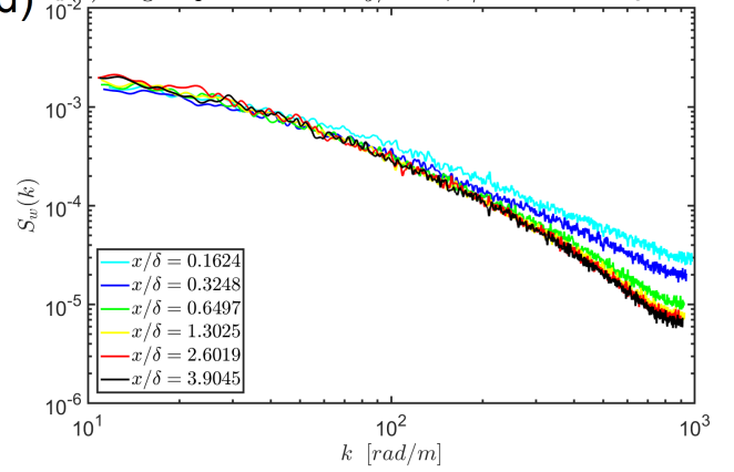
Figura 35: Grafici andamento S_u(k) e S_w(k) per le sei diverse sezioni per d_s = 3 \text{ mm} e d_s = 6 \text{ mm} , con y/\delta = 0 e z/\delta = 0.2389 . In particolare: (a) Andamento di S_u(k) per d_s = 3 \text{ mm} , (b) Andamento di S_u(k) per d_s = 6 \text{ mm} , (c) Andamento di S_w(k) per d_s = 3 \text{ mm} , (d) Andamento di S_w(k) per d_s = 6 \text{ mm}
