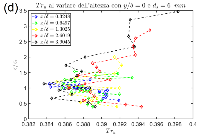
Figura 42: Grafici andamento Tr_u trasversalmente al pennacchio e al variare dell'altezza per d_s = 3 \text{ mm} e d_s = 6 \text{ mm} . In particolare: (a) Andamento di Tr_u per z/\delta = 0.2389 e d_s = 3 \text{ mm} , (b) Andamento di Tr_u per z/\delta = 0.2389 e d_s = 6 \text{ mm} , (c) Andamento di Tr_u per y/\delta = 0 e d_s = 3 \text{ mm} , (d) Andamento di Tr_u per y/\delta = 0 e d_s = 6 \text{ mm}
