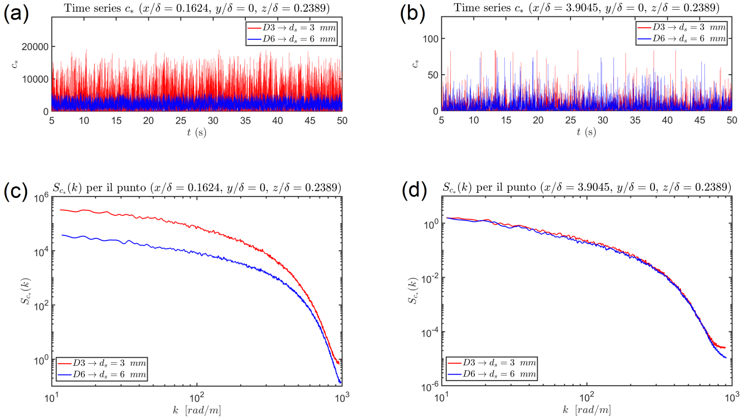
Figura 8: Confronto serie temporali di c_* con d_s = 3 mm e d_s = 6 mm misurate sull'asse del pennacchio a 51 mm e a 1226 mm dalla sorgente. In particolare: (a) Confronto serie temporali per x/\delta = 0.1624 , (b) Confronto serie temporali per x/\delta = 3.9045 , (c) Confronto spettri per x/\delta = 0.1624 , (d) Confronto spettri per x/\delta = 3.9045
