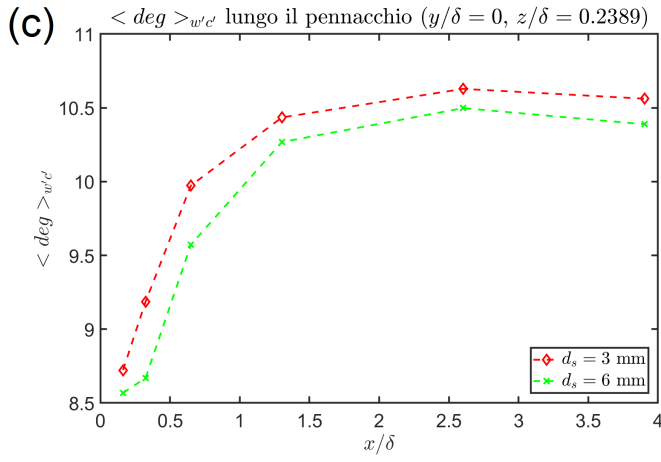
Figura 40: Grafici andamento Tr_{w'c'} , \langle d_{1n} \rangle_{w'c'} , \langle deg \rangle_{w'c'} e r_{w'c'} lungo il pennacchio, con y/\delta = 0 e z/\delta = 0.2389 ( z/z_s = 1 ). In particolare: (a) Andamento di Tr_{w'c'} , (b) Andamento di \langle d_{1n} \rangle_{w'c'} , (c) Andamento di \langle deg \rangle_{w'c'} , (d) Andamento di r_{w'c'}
