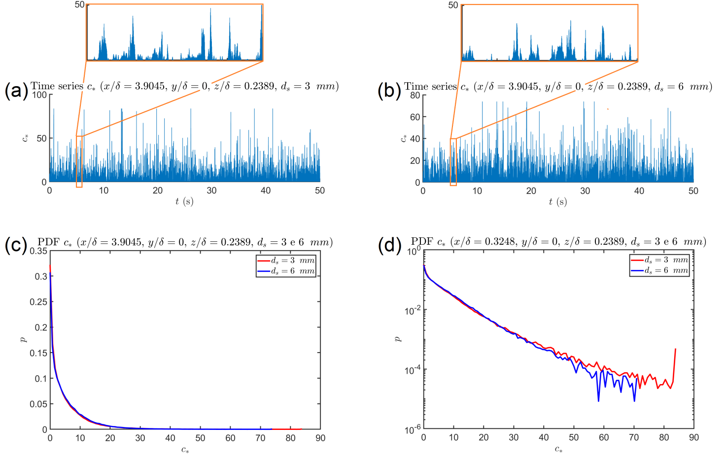
Figura 13: Grafici serie temporali e probability density functions c_* per il punto (x/\delta = 3.9045, y/\delta = 0, z/\delta = 0.2389) con d_s = 3 mm e con d_s = 6 mm. In particolare: (a) Serie temporale per d_s = 3 mm, (b) Serie temporale per d_s = 6 mm, (c) Pdf per d_s = 3 mm e per d_s = 6 mm, (d) Rappresentazione in scala semi-logaritmica delle pdf per d_s = 3 mm e per d_s = 6 mm
