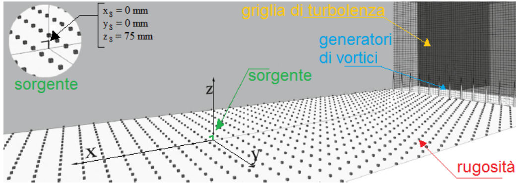
Figura 2: Rappresentazione grafica della galleria del vento con particolare della griglia di turbolenza, dei generatori di vortici, delle rugosità e della sorgente del pennacchio
