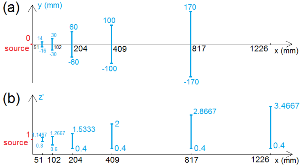
Figura 5: Rappresentazione sezioni xy e xz' e dei rispettivi intervalli di misurazione alle diverse ascisse considerate per un pennacchio con sorgente di diametro 6 millimetri
