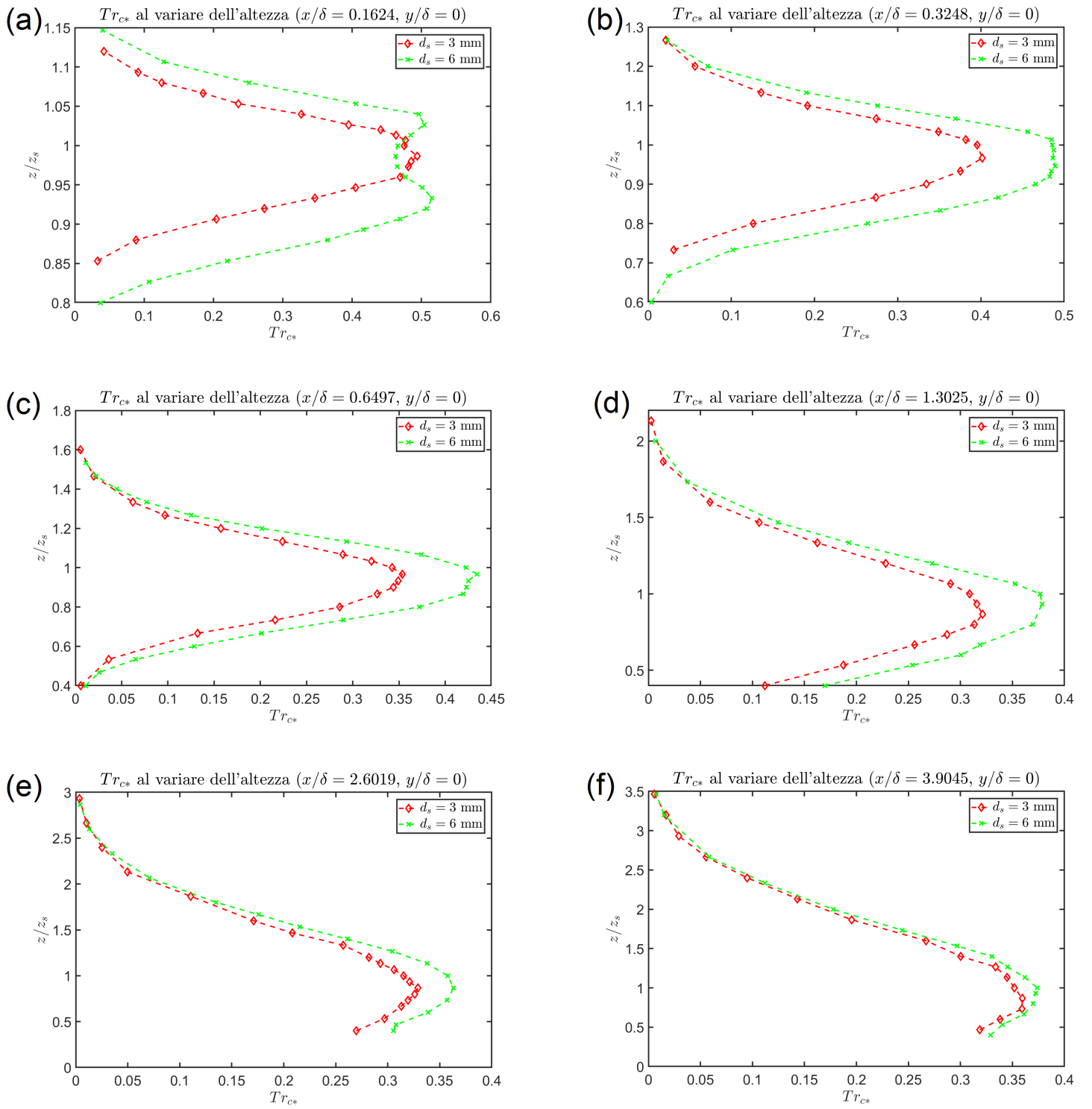
Figura 45: Grafici andamento Tr_{c*} al variare dell'altezza per le sei diverse sezioni per d_s = 3 \text{ mm} e d_s = 6 \text{ mm} , con y/\delta = 0 . In particolare: (a) Andamento di Tr_{c*} per x/\delta = 0.1624 , (b) Andamento di Tr_{c*} per x/\delta = 0.3248 , (c) Andamento di Tr_{c*} per x/\delta = 0.6497 , (d) Andamento di Tr_{c*} per x/\delta = 1.3025 , (e) Andamento di Tr_{c*} per x/\delta = 2.6019 , (f) Andamento di Tr_{c*} per x/\delta = 3.9045
