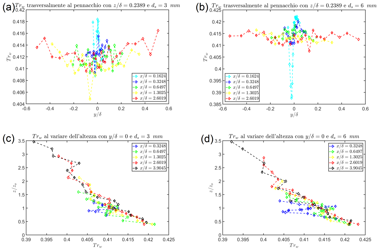
Figura 43: Grafici andamento Tr_w trasversalmente al pennacchio e al variare dell'altezza per d_s = 3 \text{ mm} e d_s = 6 \text{ mm} . In particolare: (a) Andamento di Tr_w per z/\delta = 0.2389 e d_s = 3 \text{ mm} , (b) Andamento di Tr_w per z/\delta = 0.2389 e d_s = 6 \text{ mm} , (c) Andamento di Tr_w per y/\delta = 0 e d_s = 3 \text{ mm} , (d) Andamento di Tr_w per y/\delta = 0 e d_s = 6 \text{ mm}
