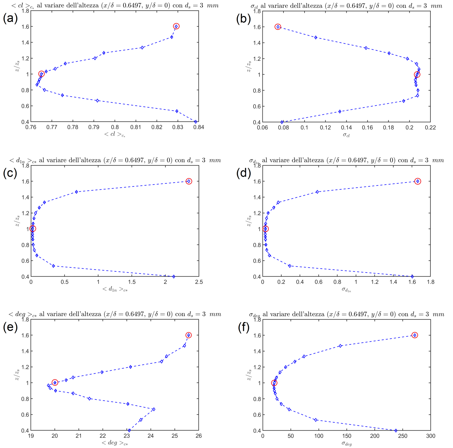
Figura 66: Grafici andamento \langle cl \rangle_{c_*} , \sigma_{cl} , \langle d_{1n} \rangle_{c_*} , \sigma_{d_{1n}} , \langle deg \rangle_{c_*} e \sigma_{deg} al variare dell'altezza, con x/\delta = 0.6497 , y/\delta = 0 e d_s = 3 \text{ mm} . In particolare: (a) Andamento di \langle cl \rangle_{c_*} , (b) Andamento di \sigma_{cl} , (c) Andamento di \langle d_{1n} \rangle_{c_*} , (d) Andamento di \sigma_{d_{1n}} , (e) Andamento di \langle deg \rangle_{c_*} , (f) Andamento di \sigma_{deg} . In rosso sono evidenziati i valori ottenuti per le due serie temporali confrontate
