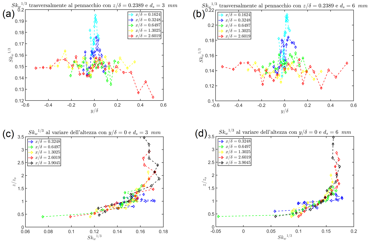
Figura 69: Grafici andamento Sk_w^{1/3} trasversalmente al pennacchio e al variare dell'altezza per d_s = 3 \text{ mm} e d_s = 6 \text{ mm} . In particolare: (a) Andamento di Sk_w^{1/3} per z/\delta = 0.2389 e d_s = 3 \text{ mm} , (b) Andamento di Sk_w^{1/3} per z/\delta = 0.2389 e d_s = 6 \text{ mm} , (c) Andamento di Sk_w^{1/3} per y/\delta = 0 e d_s = 3 \text{ mm} , (d) Andamento di Sk_w^{1/3} per y/\delta = 0 e d_s = 6 \text{ mm}
