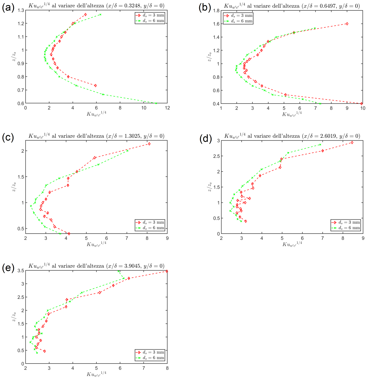
Figura 74: Grafici andamento Ku_{w'c'}^{1/4} al variare dell'altezza per le cinque diverse sezioni per d_s = 3 \text{ mm} e d_s = 6 \text{ mm} , con y/\delta = 0 . In particolare: (a) Andamento di Ku_{w'c'}^{1/4} per x/\delta = 0.3248 , (b) Andamento di Ku_{w'c'}^{1/4} per x/\delta = 0.6497 , (c) Andamento di Ku_{w'c'}^{1/4} per x/\delta = 1.3025 , (d) Andamento di Ku_{w'c'}^{1/4} per x/\delta = 2.6019 , (e) Andamento di Ku_{w'c'}^{1/4} per x/\delta = 3.9045
