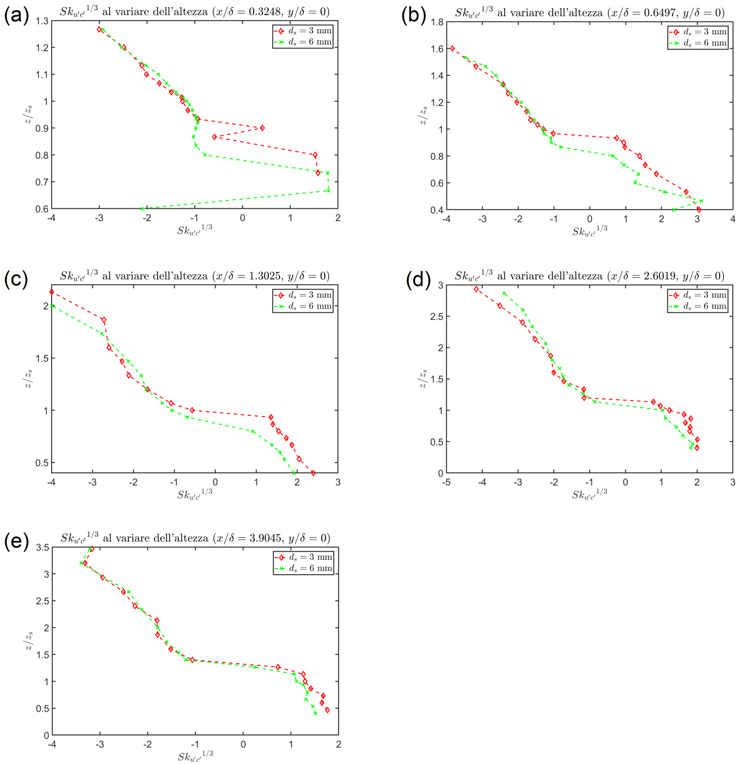
Figura 71: Grafici andamento Sk_{u'c'}^{1/3} al variare dell'altezza per le cinque diverse sezioni per d_s = 3 \text{ mm} e d_s = 6 \text{ mm} , con y/\delta = 0 . In particolare: (a) Andamento di Sk_{u'c'}^{1/3} per x/\delta = 0.3248 , (b) Andamento di Sk_{u'c'}^{1/3} per x/\delta = 0.6497 , (c) Andamento di Sk_{u'c'}^{1/3} per x/\delta = 1.3025 , (d) Andamento di Sk_{u'c'}^{1/3} per x/\delta = 2.6019 , (e) Andamento di Sk_{u'c'}^{1/3} per x/\delta = 3.9045
