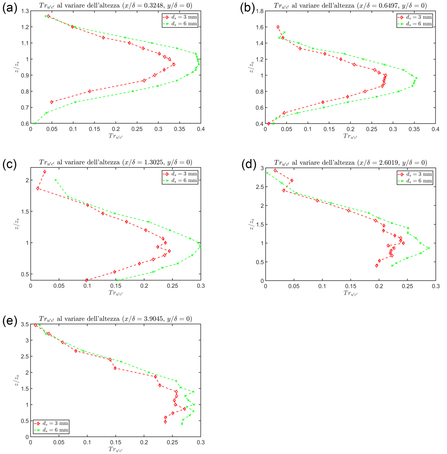
Figura 47: Grafici andamento Tr_{u'c'} al variare dell'altezza per le cinque diverse sezioni per d_s = 3 \text{ mm} e d_s = 6 \text{ mm} , con y/\delta = 0 . In particolare: (a) Andamento di Tr_{u'c'} per x/\delta = 0.3248 , (b) Andamento di Tr_{u'c'} per x/\delta = 0.6497 , (c) Andamento di Tr_{u'c'} per x/\delta = 1.3025 , (d) Andamento di Tr_{u'c'} per x/\delta = 2.6019 , (e) Andamento di Tr_{u'c'} per x/\delta = 3.9045
