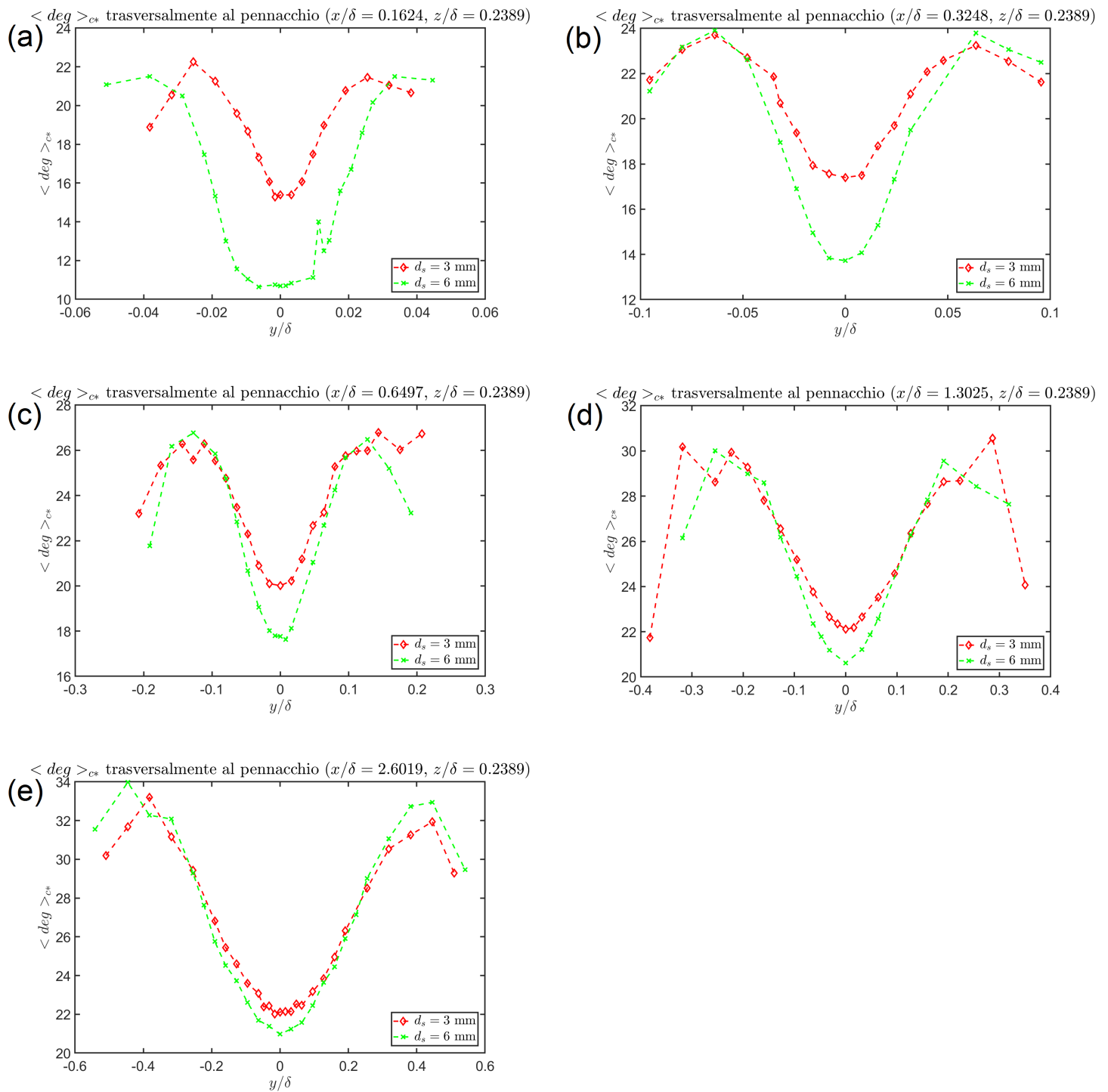
Figura 56: Grafici andamento \langle deg \rangle_{c*} trasversalmente al pennacchio per le cinque diverse sezioni per d_s = 3 \text{ mm} e d_s = 6 \text{ mm} , con z/\delta = 0.2389 ( z/z_s = 1 ). In particolare: (a) Andamento di \langle deg \rangle_{c*} per x/\delta = 0.1624 , (b) Andamento di \langle deg \rangle_{c*} per x/\delta = 0.3248 , (c) Andamento di \langle deg \rangle_{c*} per x/\delta = 0.6497 , (d) Andamento di \langle deg \rangle_{c*} per x/\delta = 1.3025 , (e) Andamento di \langle deg \rangle_{c*} per x/\delta = 2.6019
