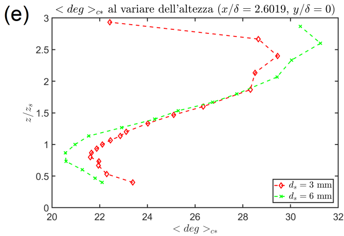
Figura 57: Grafici andamento \langle deg \rangle_{c*} al variare dell'altezza per le sei diverse sezioni per d_s = 3 \text{ mm} e d_s = 6 \text{ mm} , con y/\delta = 0 . In particolare: (a) Andamento di \langle deg \rangle_{c*} per x/\delta = 0.1624 , (b) Andamento di \langle deg \rangle_{c*} per x/\delta = 0.3248 , (c) Andamento di \langle deg \rangle_{c*} per x/\delta = 0.6497 , (d) Andamento di \langle deg \rangle_{c*} per x/\delta = 1.3025 , (e) Andamento di \langle deg \rangle_{c*} per x/\delta = 2.6019 , (f) Andamento di \langle deg \rangle_{c*} per x/\delta = 3.9045
