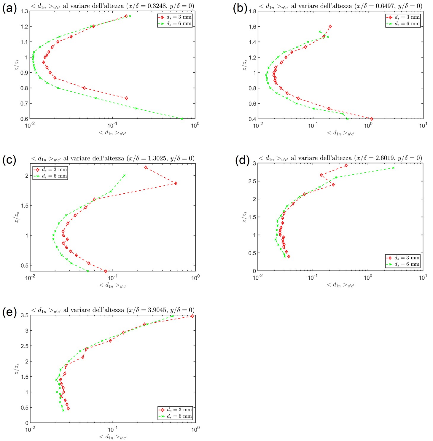
Figura 53: Grafici andamento \langle d_{1n} \rangle_{u'c'} al variare dell'altezza per le cinque diverse sezioni per d_s = 3 \text{ mm} e d_s = 6 \text{ mm} , con y/\delta = 0 . In particolare: (a) Andamento di \langle d_{1n} \rangle_{u'c'} per x/\delta = 0.3248 , (b) Andamento di \langle d_{1n} \rangle_{u'c'} per x/\delta = 0.6497 , (c) Andamento di \langle d_{1n} \rangle_{u'c'} per x/\delta = 1.3025 , (d) Andamento di \langle d_{1n} \rangle_{u'c'} per x/\delta = 2.6019 , (e) Andamento di \langle d_{1n} \rangle_{u'c'} per x/\delta = 3.9045
