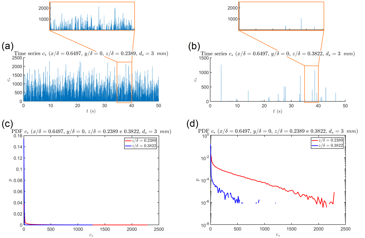
Figura 67: Grafici serie temporali e probability density functions c_* per i punti (x/\delta = 0.6497, y/\delta = 0, z/\delta = 0.2389) e (x/\delta = 0.6497, y/\delta = 0, z/\delta = 0.3822) con d_s = 3 \text{ mm} . In particolare: (a) Serie temporale per z/\delta = 0.2389 , (b) Serie temporale per z/\delta = 0.3822 , (c) Pdf per z/\delta = 0.2389 e per z/\delta = 0.3822 , (d) Rappresentazione in scala semi-logaritmica della pdf per z/\delta = 0.2389 e per z/\delta = 0.3822
