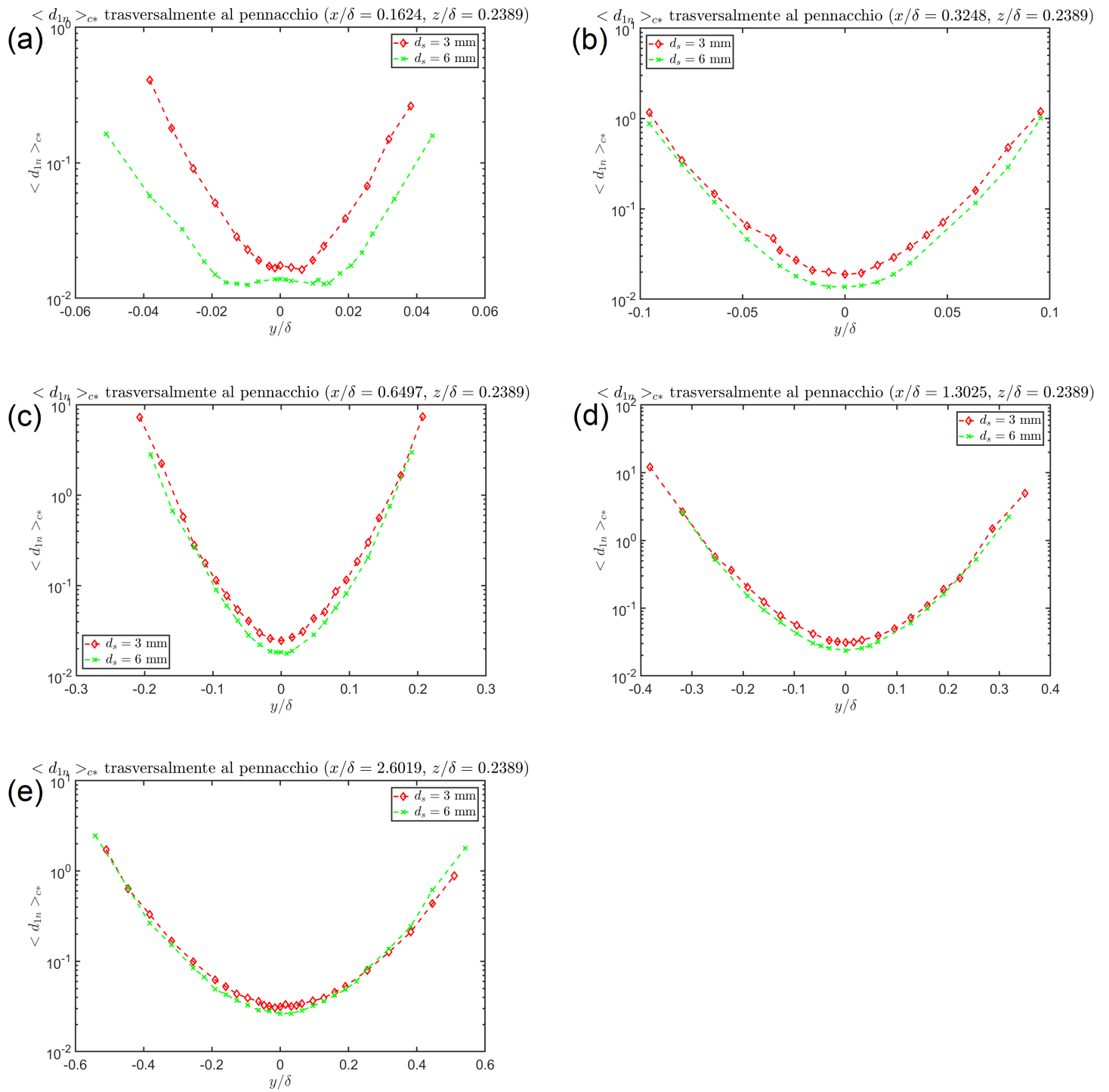
Figura 50: Grafici andamento \langle d_{1n} \rangle_{c^*} trasversalmente al pennacchio per le cinque diverse sezioni per d_s = 3\text{ mm} e d_s = 6\text{ mm} , con z/\delta = 0.2389 ( z/z_s = 1 ). In particolare: (a) Andamento di \langle d_{1n} \rangle_{c^*} per x/\delta = 0.1624 , (b) Andamento di \langle d_{1n} \rangle_{c^*} per x/\delta = 0.3248 , (c) Andamento di \langle d_{1n} \rangle_{c^*} per x/\delta = 0.6497 , (d) Andamento di \langle d_{1n} \rangle_{c^*} per x/\delta = 1.3025 , (e) Andamento di \langle d_{1n} \rangle_{c^*} per x/\delta = 2.6019
