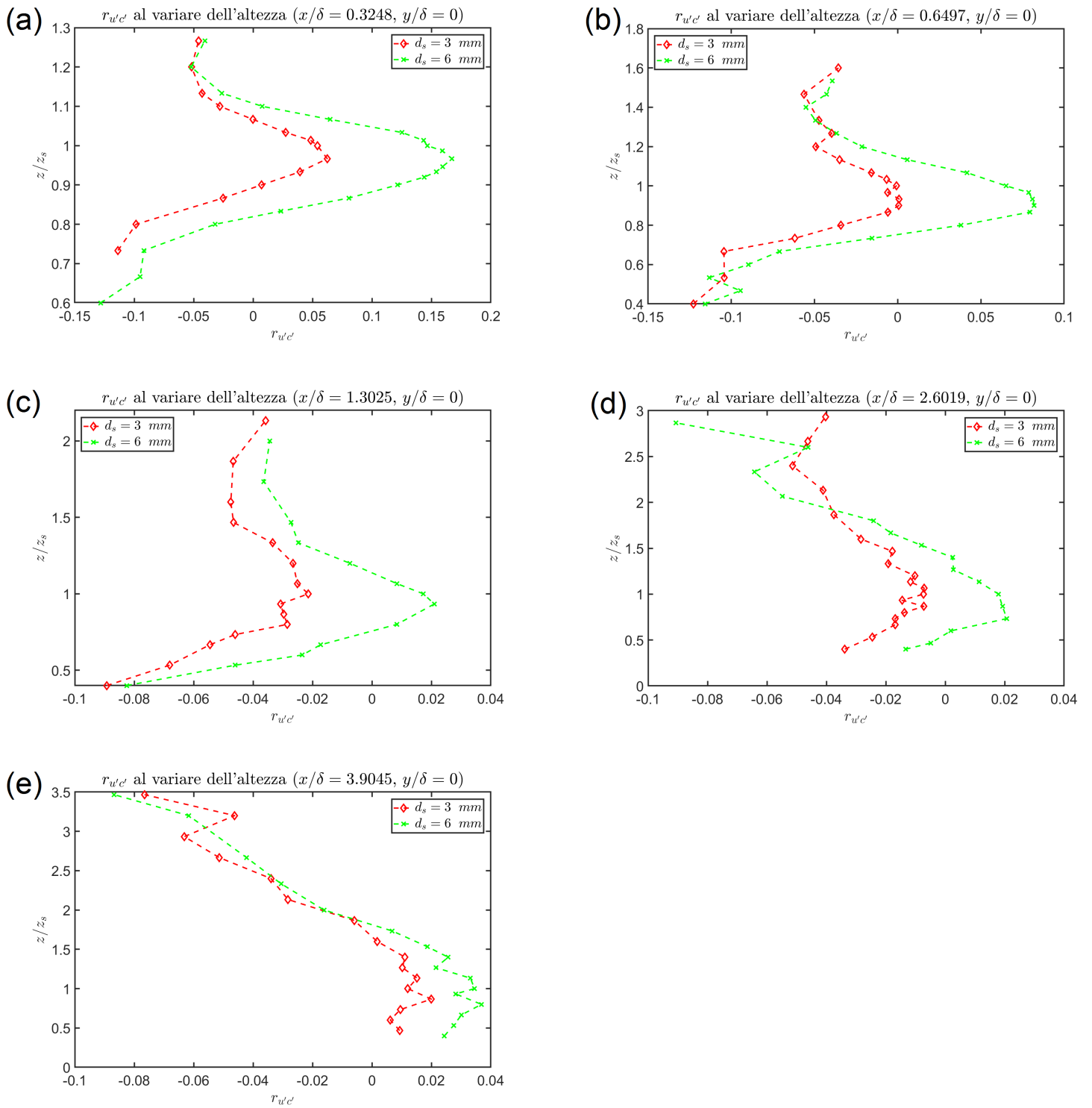
Figura 65: Grafici andamento r_{u'c'} al variare dell'altezza per le cinque diverse sezioni per d_s = 3 mm e d_s = 6 mm, con y/\delta = 0 . In particolare: (a) Andamento di r_{u'c'} per x/\delta = 0.3248 , (b) Andamento di r_{u'c'} per x/\delta = 0.6497 , (c) Andamento di r_{u'c'} per x/\delta = 1.3025 , (d) Andamento di r_{u'c'} per x/\delta = 2.6019 , (e) Andamento di r_{u'c'} per x/\delta = 3.9045
