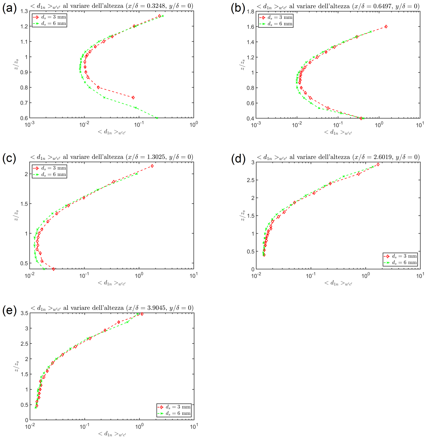
Figura 52: Grafici andamento \langle d_{1n} \rangle_{w'c'} al variare dell'altezza per le cinque diverse sezioni per d_s = 3 \text{ mm} e d_s = 6 \text{ mm} , con y/\delta = 0 . In particolare: (a) Andamento di \langle d_{1n} \rangle_{w'c'} per x/\delta = 0.3248 , (b) Andamento di \langle d_{1n} \rangle_{w'c'} per x/\delta = 0.6497 , (c) Andamento di \langle d_{1n} \rangle_{w'c'} per x/\delta = 1.3025 , (d) Andamento di \langle d_{1n} \rangle_{w'c'} per x/\delta = 2.6019 , (e) Andamento di \langle d_{1n} \rangle_{w'c'} per x/\delta = 3.9045
