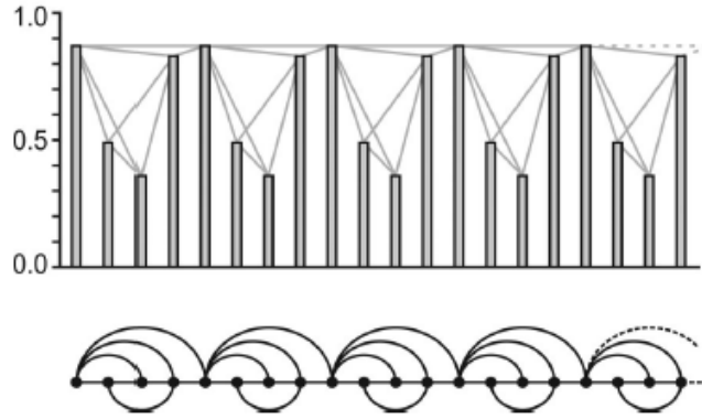
Figura 9: Rappresentazione della costruzione del visibility graph
