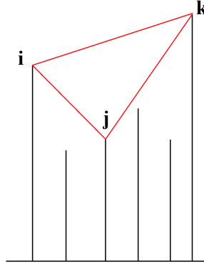
Figura 10: Triangolo formato tra i nodi della terna (i, j, k)
