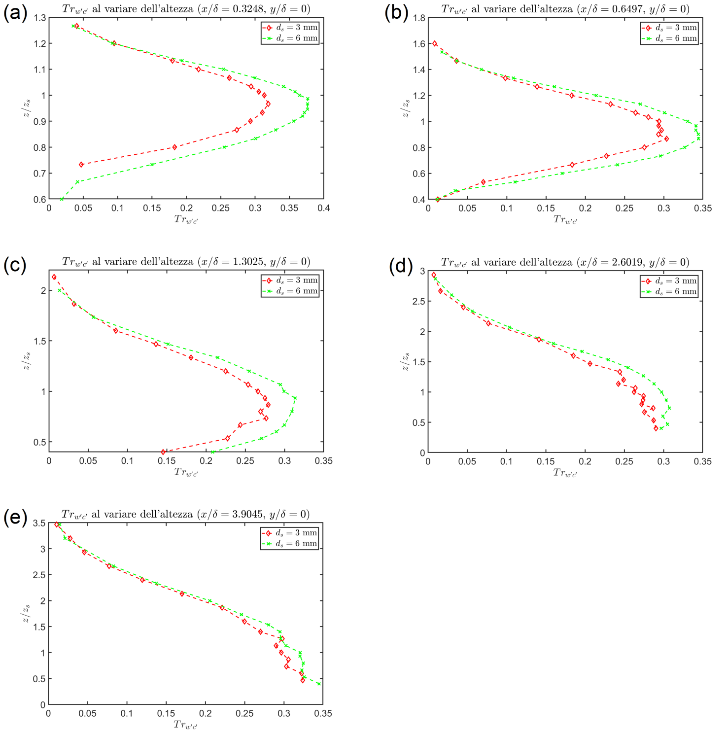
Figura 46: Grafici andamento Tr_{w'c'} al variare dell'altezza per le cinque diverse sezioni per d_s = 3 \text{ mm} e d_s = 6 \text{ mm} , con y/\delta = 0 . In particolare: (a) Andamento di Tr_{w'c'} per x/\delta = 0.3248 , (b) Andamento di Tr_{w'c'} per x/\delta = 0.6497 , (c) Andamento di Tr_{w'c'} per x/\delta = 1.3025 , (d) Andamento di Tr_{w'c'} per x/\delta = 2.6019 , (e) Andamento di Tr_{w'c'} per x/\delta = 3.9045
