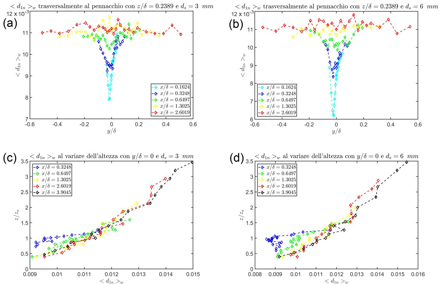
Figura 49: Grafici andamento \langle d_{1n} \rangle_w trasversalmente al pennacchio e al variare dell'altezza per d_s = 3 \text{ mm} e d_s = 6 \text{ mm} . In particolare: (a) Andamento di \langle d_{1n} \rangle_w per z/\delta = 0.2389 e d_s = 3 \text{ mm} , (b) Andamento di \langle d_{1n} \rangle_w per z/\delta = 0.2389 e d_s = 6 \text{ mm} , (c) Andamento di \langle d_{1n} \rangle_w per y/\delta = 0 e d_s = 3 \text{ mm} , (d) Andamento di \langle d_{1n} \rangle_w per y/\delta = 0 e d_s = 6 \text{ mm}
