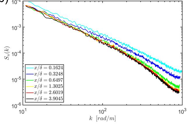
(b) S_u(k) lungo il pennacchio con y/\delta = 0 , z/\delta = 0.2389 e d_s = 6 \text{ mm}
