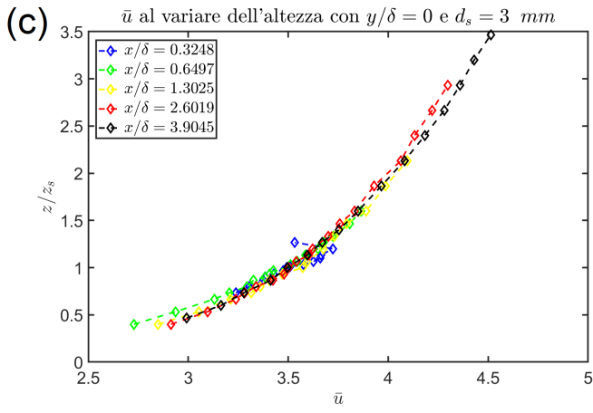
Figura 18: Grafici andamento \bar{u} trasversalmente al pennacchio e al variare dell'altezza per d_s = 3 \text{ mm} e d_s = 6 \text{ mm} . In particolare: (a) Andamento di \bar{u} per z/\delta = 0.2389 e d_s = 3 \text{ mm} , (b) Andamento di \bar{u} per z/\delta = 0.2389 e d_s = 6 \text{ mm} , (c) Andamento di \bar{u} per y/\delta = 0 e d_s = 3 \text{ mm} , (d) Andamento di \bar{u} per y/\delta = 0 e d_s = 6 \text{ mm}
