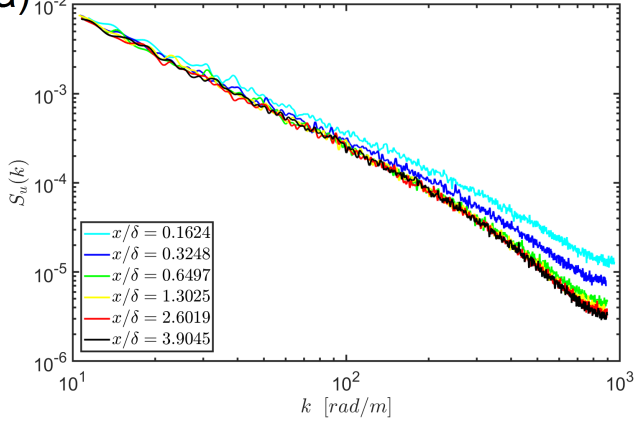
(a) S_u(k) lungo il pennacchio con y/\delta = 0 , z/\delta = 0.2389 e d_s = 3 \text{ mm}
