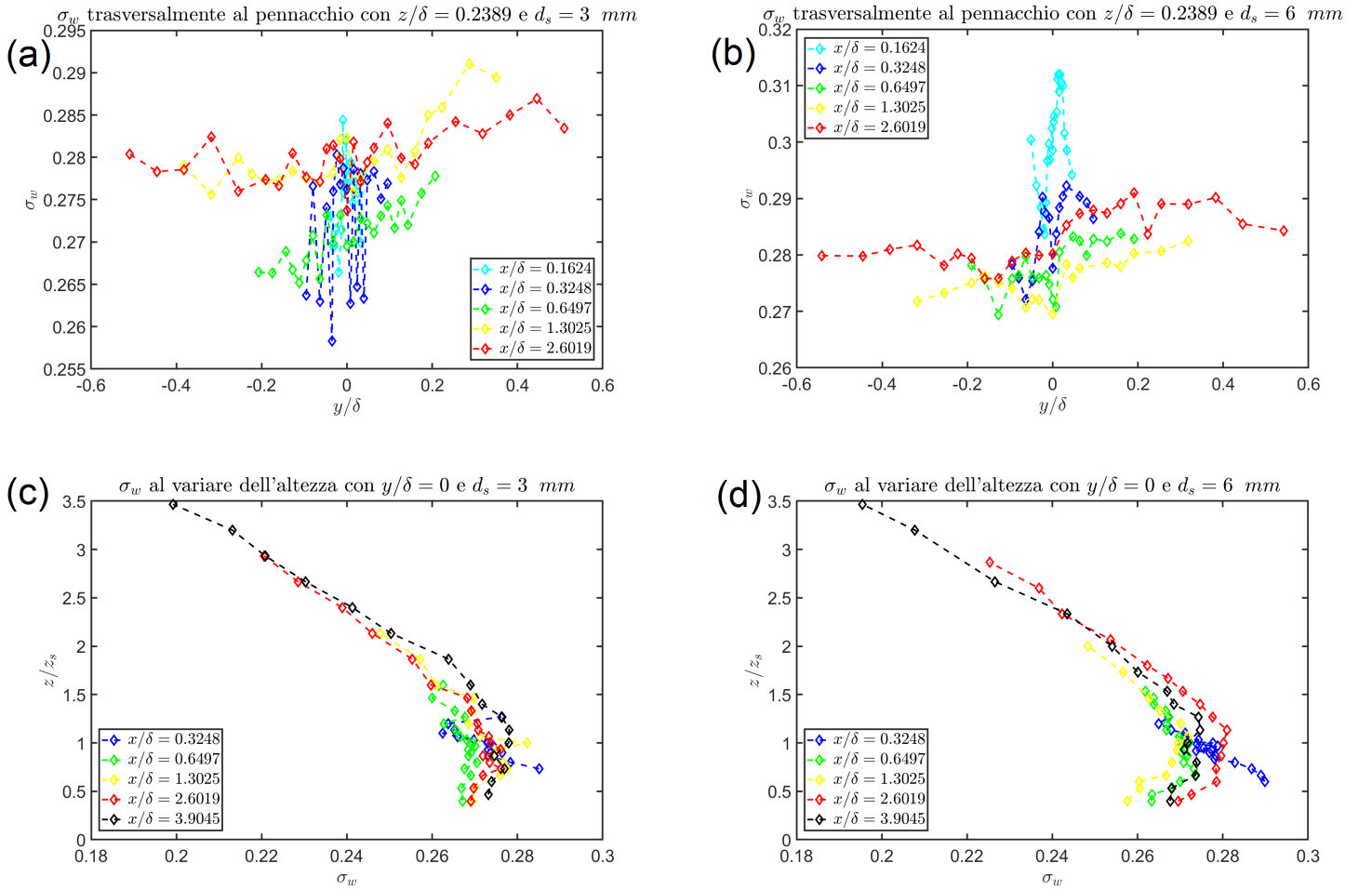
Figura 25: Grafici andamento \sigma_w trasversalmente al pennacchio e al variare dell'altezza per d_s = 3 mm e d_s = 6 mm. In particolare: (a) Andamento di \sigma_w per z/\delta = 0.2389 e d_s = 3 mm, (b) Andamento di \sigma_w per z/\delta = 0.2389 e d_s = 6 mm, (c) Andamento di \sigma_w per y/\delta = 0 e d_s = 3 mm, (d) Andamento di \sigma_w per y/\delta = 0 e d_s = 6 mm
