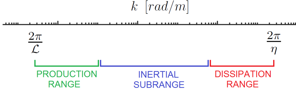
Figura 6: Rappresentazione grafica dei tre range in cui è suddiviso lo spazio dei numeri d'onda
