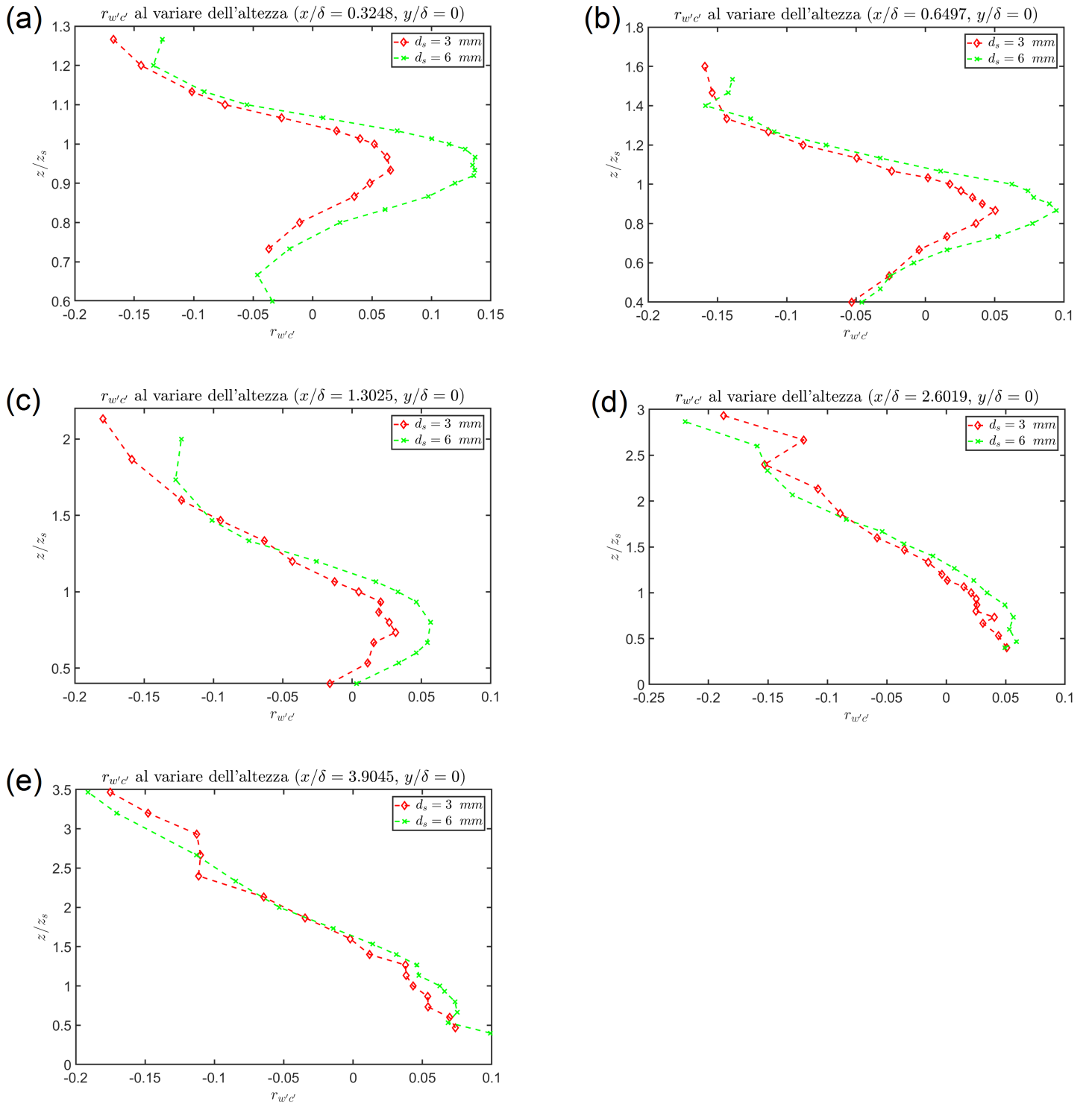
Figura 64: Grafici andamento r_{w'c'} al variare dell'altezza per le cinque diverse sezioni per d_s = 3 \text{ mm} e d_s = 6 \text{ mm} , con y/\delta = 0 . In particolare: (a) Andamento di r_{w'c'} per x/\delta = 0.3248 , (b) Andamento di r_{w'c'} per x/\delta = 0.6497 , (c) Andamento di r_{w'c'} per x/\delta = 1.3025 , (d) Andamento di r_{w'c'} per x/\delta = 2.6019 , (e) Andamento di r_{w'c'} per x/\delta = 3.9045
