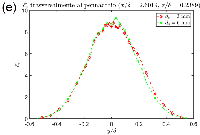
Figura 20: Grafici andamento \bar{c}_* trasversalmente al pennacchio per le cinque diverse sezioni per d_s = 3 \text{ mm} e d_s = 6 \text{ mm} , con z/z_s = 0.2389 ( z/z_s = 1 ). In particolare: (a) Andamento di \bar{c}_* per x/\delta = 0.1624 , (b) Andamento di \bar{c}_* per x/\delta = 0.3248 , (c) Andamento di \bar{c}_* per x/\delta = 0.6497 , (d) Andamento di \bar{c}_* per x/\delta = 1.3025 , (e) Andamento di \bar{c}_* per x/\delta = 2.6019
