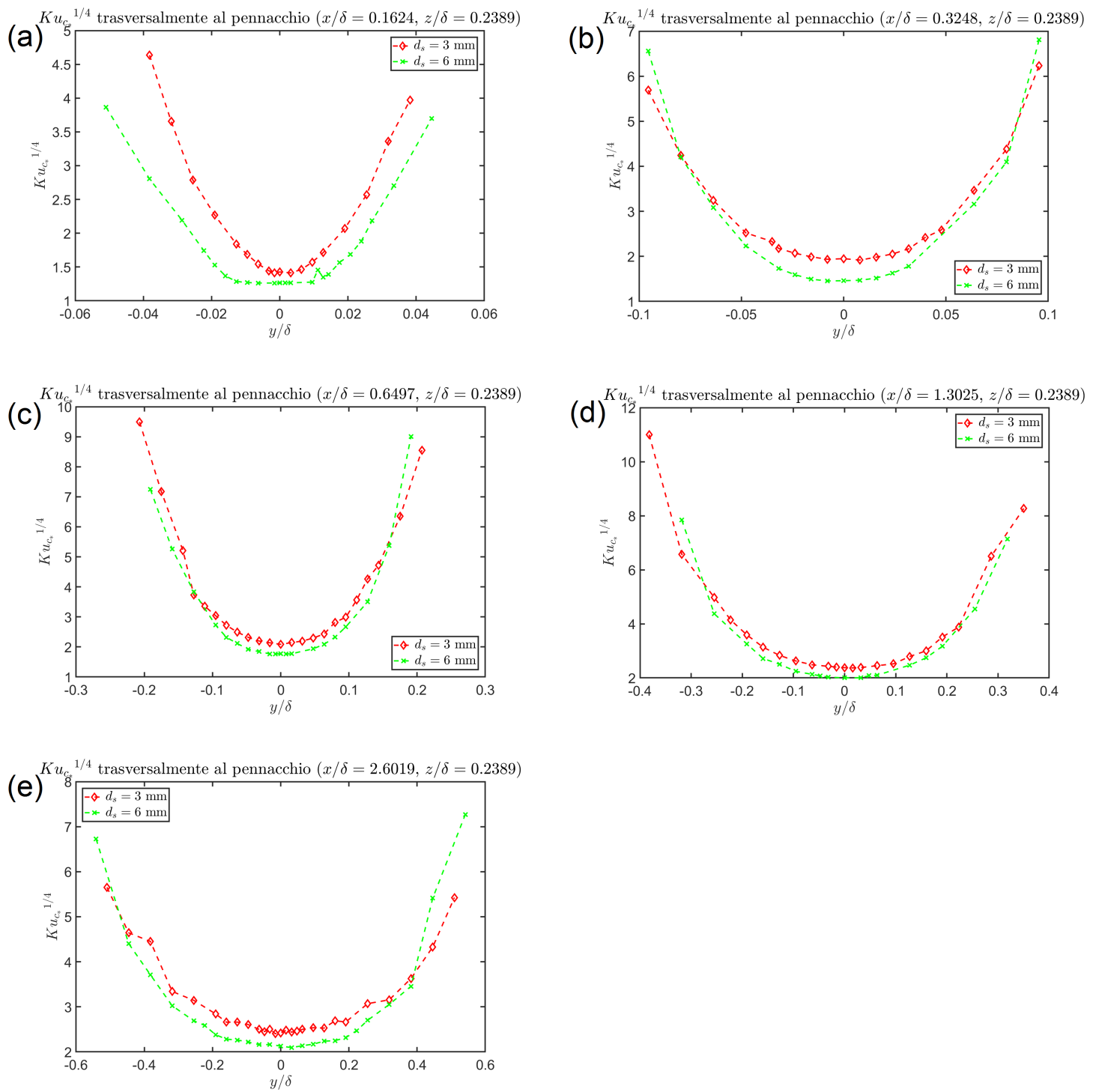
Figura 32: Grafici andamento Ku_{c_*}^{1/4} trasversalmente al pennacchio per le cinque diverse sezioni per d_s = 3 mm e d_s = 6 mm, con z/\delta = 0.2389 ( z/z_s = 1 ). In particolare: (a) Andamento di Ku_{c_*}^{1/4} per x/\delta = 0.1624 , (b) Andamento di Ku_{c_*}^{1/4} per x/\delta = 0.3248 , (c) Andamento di Ku_{c_*}^{1/4} per x/\delta = 0.6497 , (d) Andamento di Ku_{c_*}^{1/4} per x/\delta = 1.3025 , (e) Andamento di Ku_{c_*}^{1/4} per x/\delta = 2.6019
