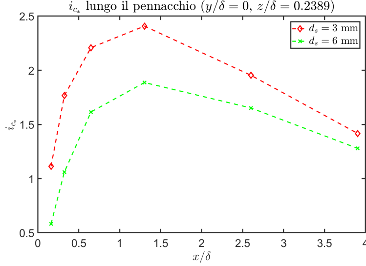
Figura 15: Grafico andamento intensità delle fluttuazioni di concentrazione lungo il pennacchio
