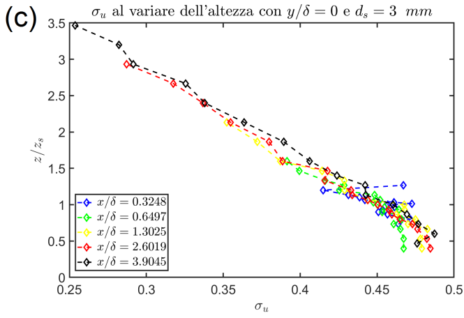
Figura 24: Grafici andamento \sigma_u trasversalmente al pennacchio e al variare dell'altezza per d_s = 3 \text{ mm} e d_s = 6 \text{ mm} . In particolare: (a) Andamento di \sigma_u per z/\delta = 0.2389 e d_s = 3 \text{ mm} , (b) Andamento di \sigma_u per z/\delta = 0.2389 e d_s = 6 \text{ mm} , (c) Andamento di \sigma_u per y/\delta = 0 e d_s = 3 \text{ mm} , (d) Andamento di \sigma_u per y/\delta = 0 e d_s = 6 \text{ mm}
