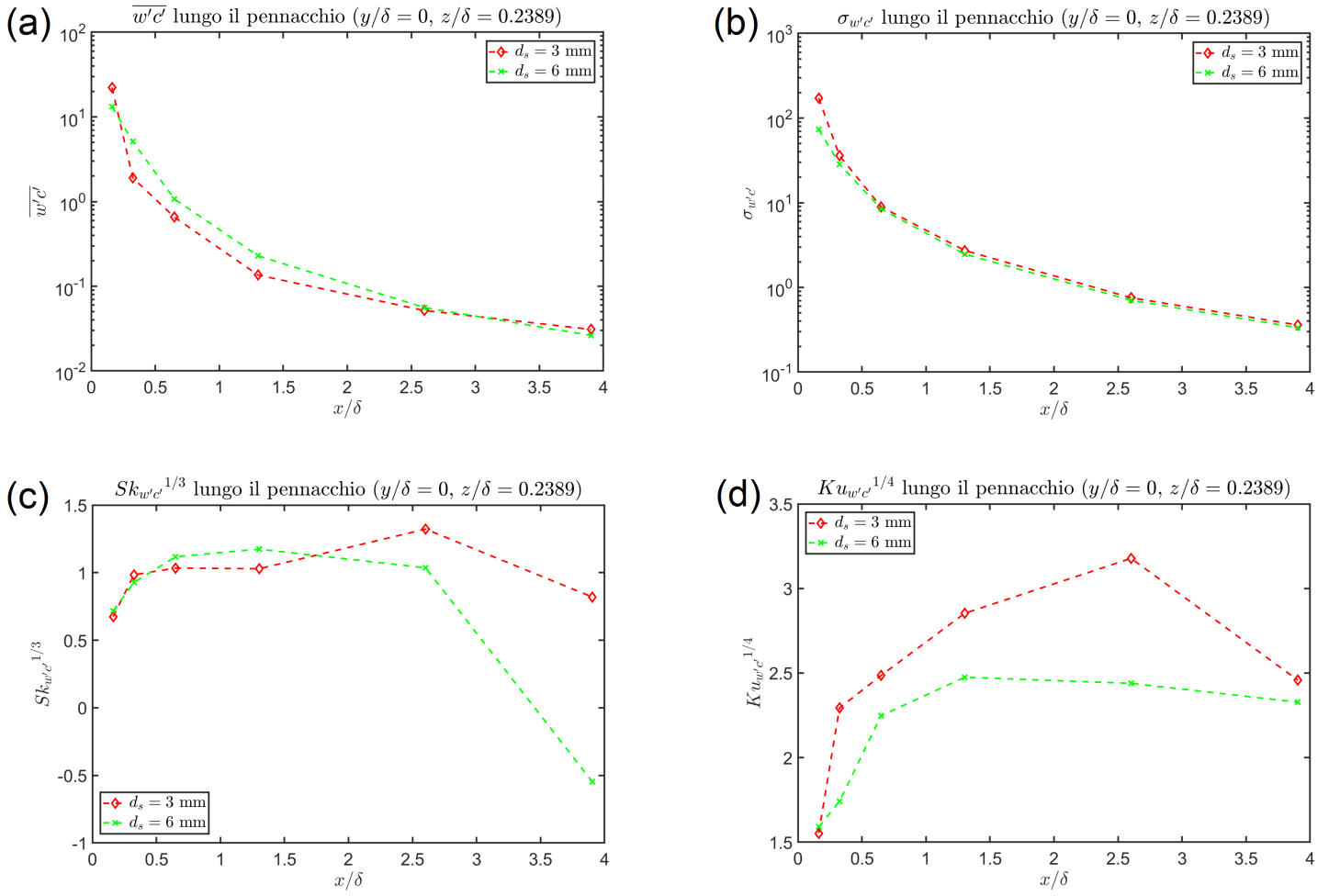
Figura 16: Grafici andamento \overline{w'c'} , \sigma_{w'c'} , Sk_{w'c'}^{1/3} e Ku_{w'c'}^{1/4} lungo il pennacchio, con y/\delta = 0 e z/\delta = 0.2389 ( z/z_s = 1 ). In particolare: (a) Andamento di \overline{w'c'} in scala semi-logaritmica, (b) Andamento di \sigma_{w'c'} in scala semi-logaritmica, (c) Andamento di Sk_{w'c'}^{1/3} , (d) Andamento di Ku_{w'c'}^{1/4}
