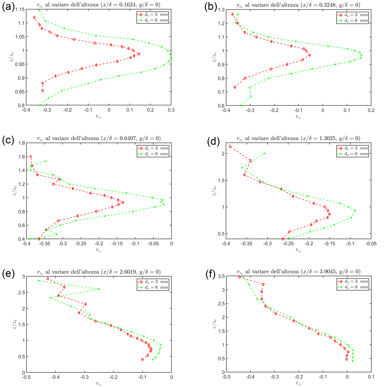
Figura 63: Grafici andamento r_{c*} al variare dell'altezza per le sei diverse sezioni per d_s = 3 \text{ mm} e d_s = 6 \text{ mm} , con z/\delta = 0.2389 ( z/z_s = 1 ). In particolare: (a) Andamento di r_{c*} per x/\delta = 0.1624 , (b) Andamento di r_{c*} per x/\delta = 0.3248 , (c) Andamento di r_{c*} per x/\delta = 0.6497 , (d) Andamento di r_{c*} per x/\delta = 1.3025 , (e) Andamento di r_{c*} per x/\delta = 2.6019 , (f) Andamento di r_{c*} per x/\delta = 3.9045
