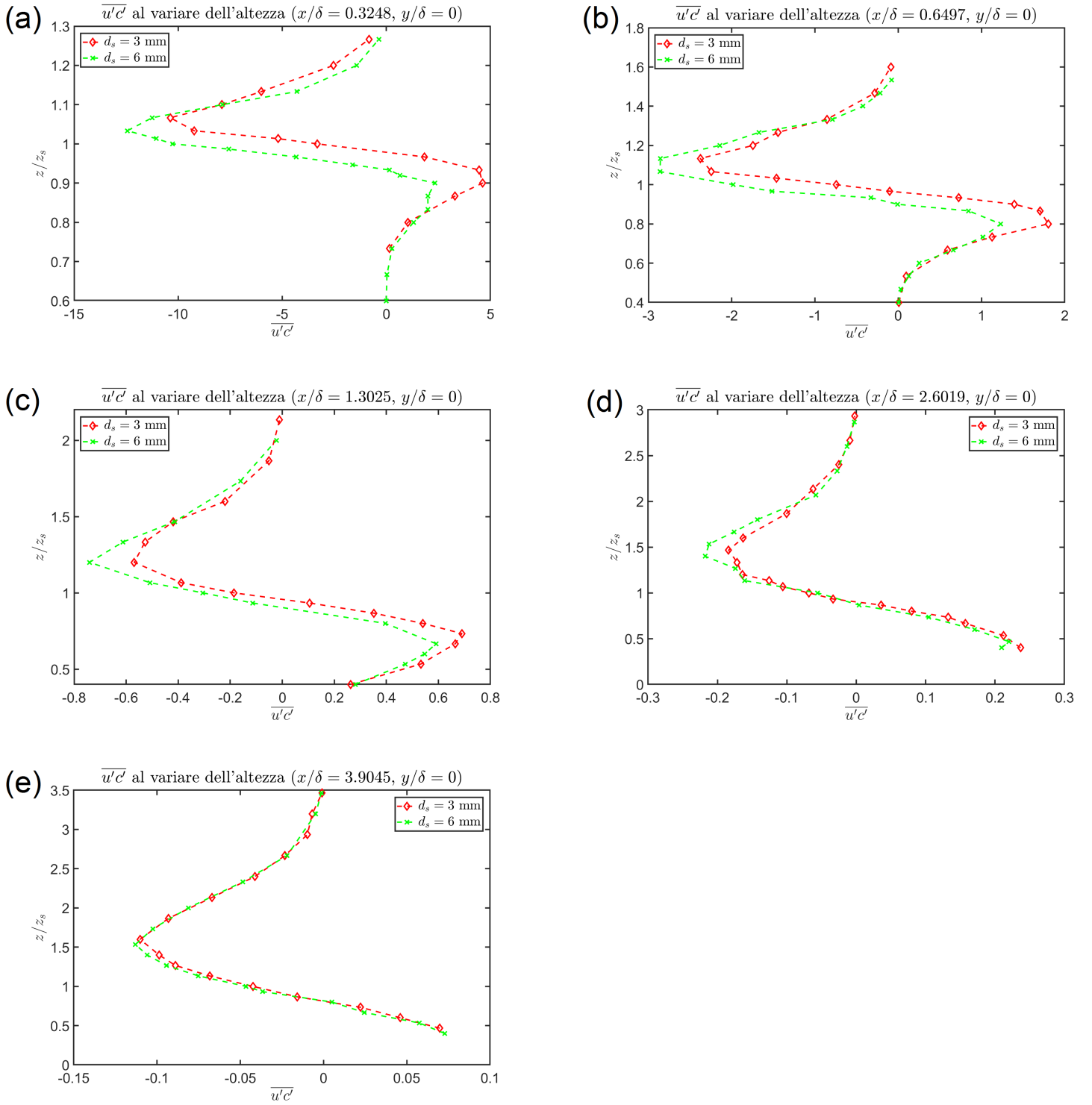
Figura 23: Grafici andamento \overline{u'c'} al variare dell'altezza per le cinque diverse sezioni per d_s = 3 \text{ mm} e d_s = 6 \text{ mm} , con y/\delta = 0 . In particolare: (a) Andamento di \overline{u'c'} per x/\delta = 0.3248 , (b) Andamento di \overline{u'c'} per x/\delta = 0.6497 , (c) Andamento di \overline{u'c'} per x/\delta = 1.3025 , (d) Andamento di \overline{u'c'} per x/\delta = 2.6019 , (e) Andamento di \overline{u'c'} per x/\delta = 3.9045
