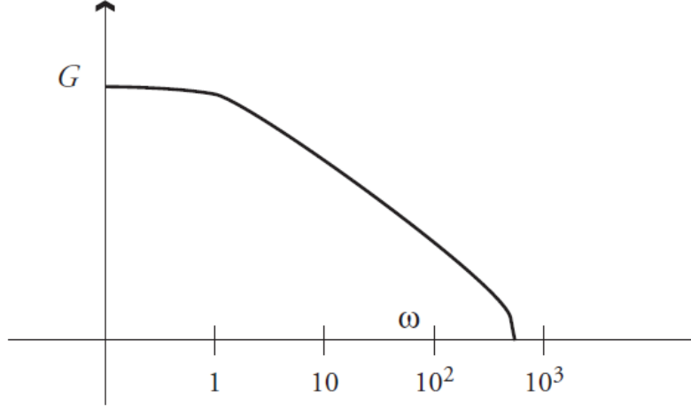
Figura 7: Grafico dell'andamento atteso dello spettro di potenza G(\omega) al variare della pulsazione \omega
