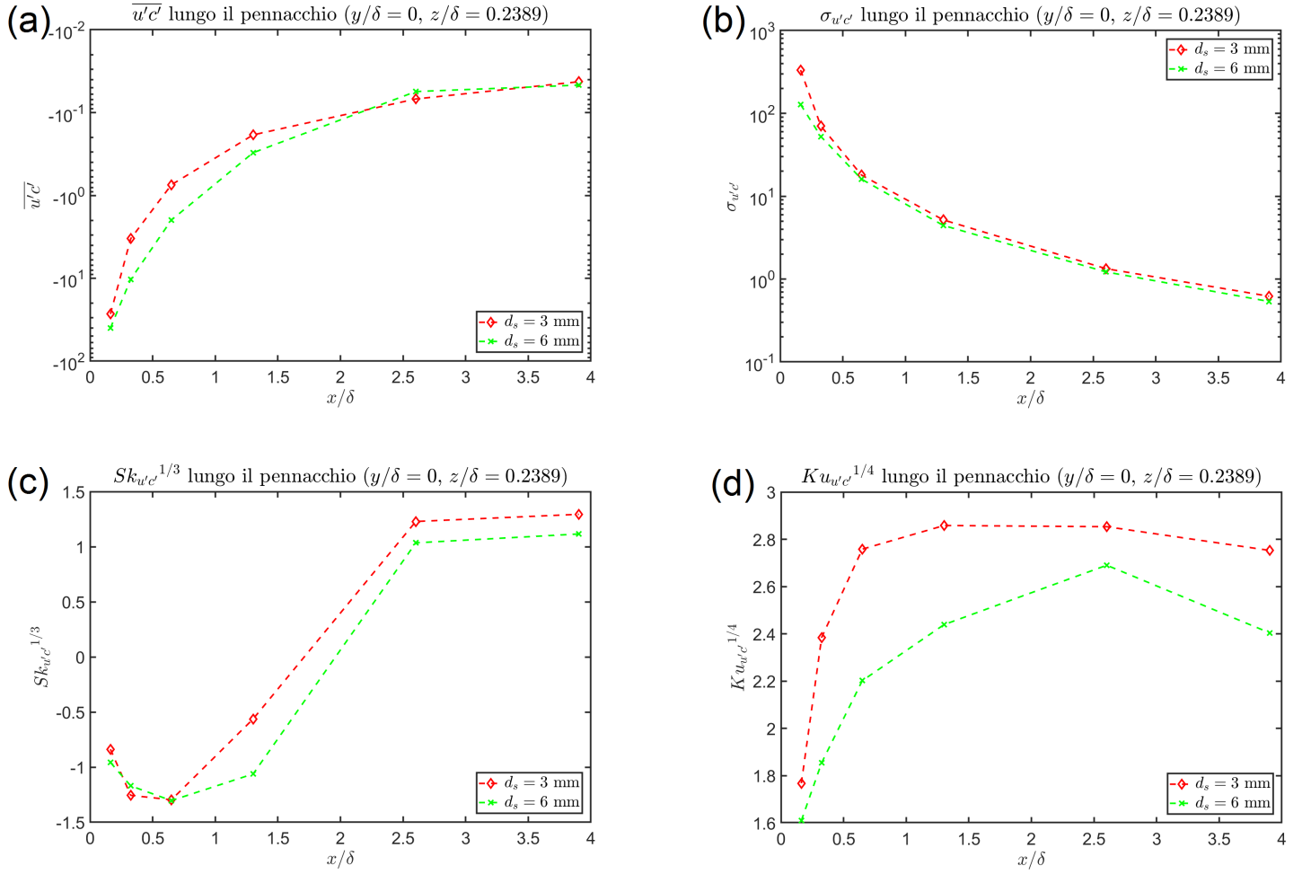
Figura 17: Grafici andamento \overline{u'c'} , \sigma_{u'c'} , Sk_{u'c'}^{1/3} e Ku_{u'c'}^{1/4} lungo il pennacchio, con y/\delta = 0 e z/\delta = 0.2389 ( z/z_s = 1 ). In particolare: (a) Andamento di \overline{u'c'} in scala semi-logaritmica, (b) Andamento di \sigma_{u'c'} in scala semi-logaritmica, (c) Andamento di Sk_{u'c'}^{1/3} , (d) Andamento di Ku_{u'c'}^{1/4}
