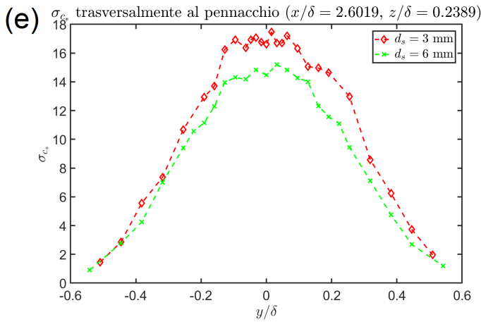
Figura 26: Grafici andamento \sigma_{c_*} trasversalmente al pennacchio per le cinque diverse sezioni per d_s = 3 \text{ mm} e d_s = 6 \text{ mm} , con z/\delta = 0.2389 ( z/z_s = 1 ). In particolare: (a) Andamento di \sigma_{c_*} per x/\delta = 0.1624 , (b) Andamento di \sigma_{c_*} per x/\delta = 0.3248 , (c) Andamento di \sigma_{c_*} per x/\delta = 0.6497 , (d) Andamento di \sigma_{c_*} per x/\delta = 1.3025 , (e) Andamento di \sigma_{c_*} per x/\delta = 2.6019
