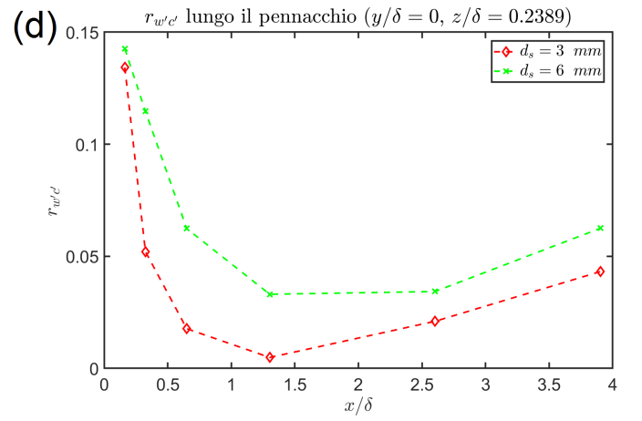
Figura 40: Grafici andamento Tr_{w'c'} , \langle d_{1n} \rangle_{w'c'} , \langle deg \rangle_{w'c'} e r_{w'c'} lungo il pennacchio, con y/\delta = 0 e z/\delta = 0.2389 ( z/z_s = 1 ). In particolare: (a) Andamento di Tr_{w'c'} , (b) Andamento di \langle d_{1n} \rangle_{w'c'} , (c) Andamento di \langle deg \rangle_{w'c'} , (d) Andamento di r_{w'c'}
