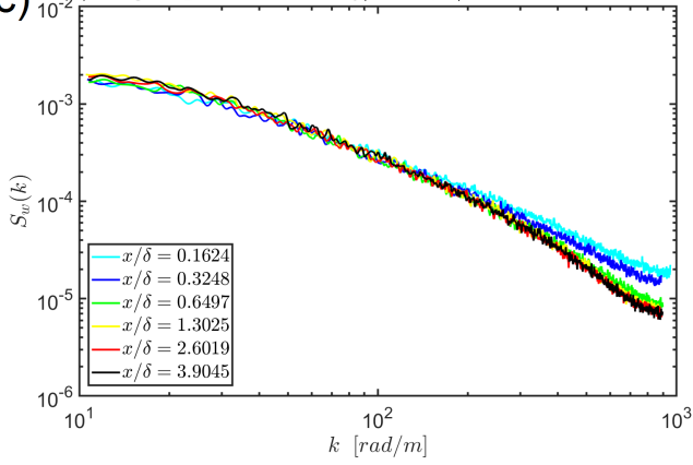
Figura 35: Grafici andamento S_u(k) e S_w(k) per le sei diverse sezioni per d_s = 3 \text{ mm} e d_s = 6 \text{ mm} , con y/\delta = 0 e z/\delta = 0.2389 . In particolare: (a) Andamento di S_u(k) per d_s = 3 \text{ mm} , (b) Andamento di S_u(k) per d_s = 6 \text{ mm} , (c) Andamento di S_w(k) per d_s = 3 \text{ mm} , (d) Andamento di S_w(k) per d_s = 6 \text{ mm}
