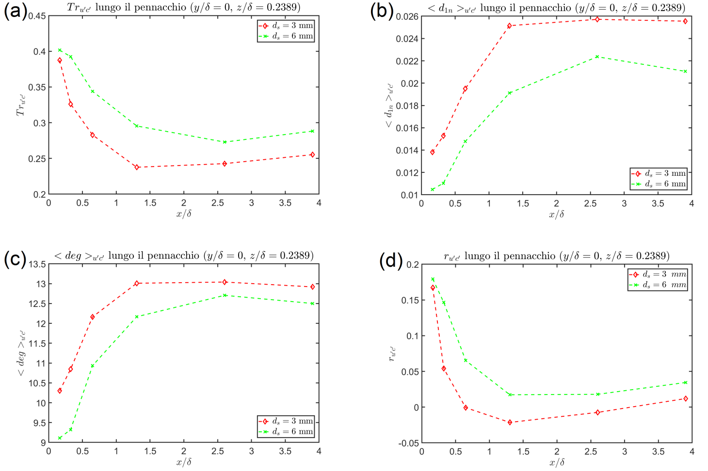
Figura 41: Grafici andamento Tr_{u'c'} , \langle d_{1n} \rangle_{u'c'} , \langle deg \rangle_{u'c'} e r_{u'c'} lungo il pennacchio, con y/\delta = 0 e z/\delta = 0.2389 ( z/z_s = 1 ). In particolare: (a) Andamento di Tr_{u'c'} , (b) Andamento di \langle d_{1n} \rangle_{u'c'} , (c) Andamento di \langle deg \rangle_{u'c'} , (d) Andamento di r_{u'c'}
