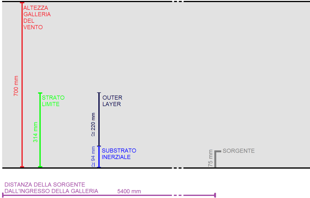
Figura 3: Sezione verticale della galleria del vento con particolare delle diverse regioni in cui è suddiviso il campo di moto
