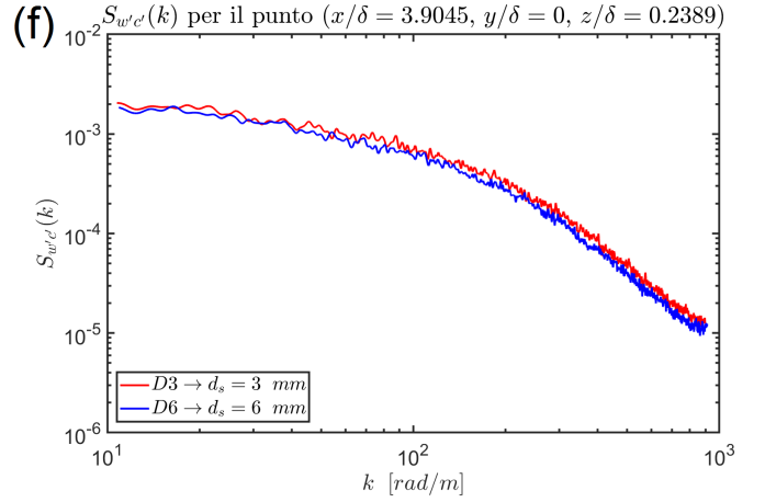
Figura 37: Grafici andamento S_{w'c'}(k) per le sei diverse sezioni per d_s = 3 \text{ mm} e d_s = 6 \text{ mm} , con y/\delta = 0 e z/\delta = 0.2389 . In particolare: (a) Andamento di S_{w'c'}(k) per x/\delta = 0.1624 , (b) Andamento di S_{w'c'}(k) per x/\delta = 0.3248 , (c) Andamento di S_{w'c'}(k) per x/\delta = 0.6497 , (d) Andamento di S_{w'c'}(k) per x/\delta = 1.3025 , (e) Andamento di S_{w'c'}(k) per x/\delta = 2.6019 , (f) Andamento di S_{w'c'}(k) per x/\delta = 3.9045
