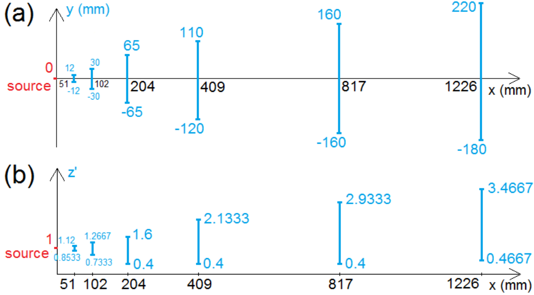
Figura 4: Rappresentazione sezioni xy e xz' e dei rispettivi intervalli di misurazione alle diverse ascisse considerate per un pennacchio con sorgente di diametro 3 millimetri
