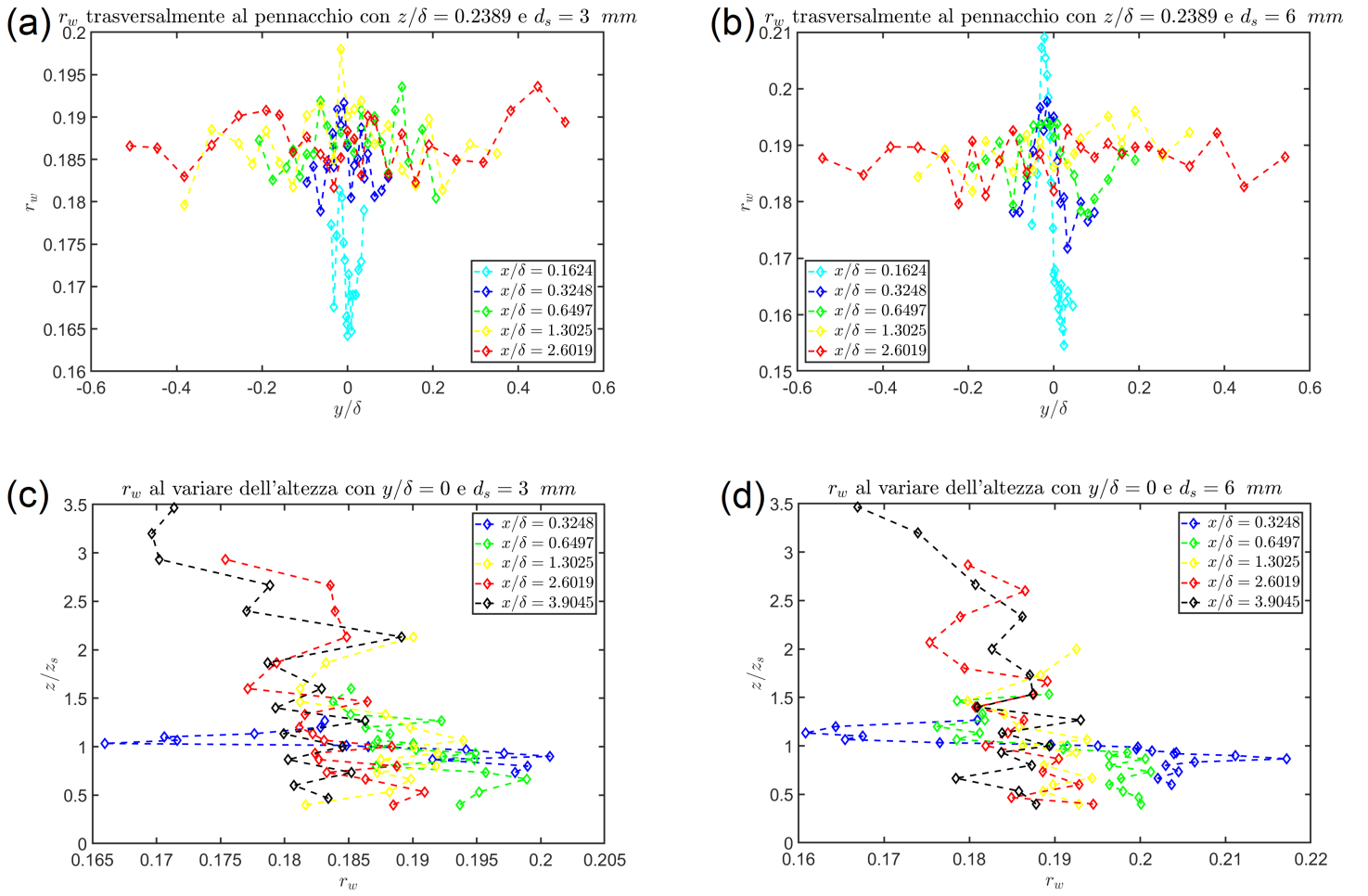
Figura 61: Grafici andamento r_w trasversalmente al pennacchio e al variare dell'altezza per d_s = 3 \text{ mm} e d_s = 6 \text{ mm} . In particolare: (a) Andamento di r_w per z/\delta = 0.2389 e d_s = 3 \text{ mm} , (b) Andamento di r_w per z/\delta = 0.2389 e d_s = 6 \text{ mm} , (c) Andamento di r_w per y/\delta = 0 e d_s = 3 \text{ mm} , (d) Andamento di r_w per y/\delta = 0 e d_s = 6 \text{ mm}
