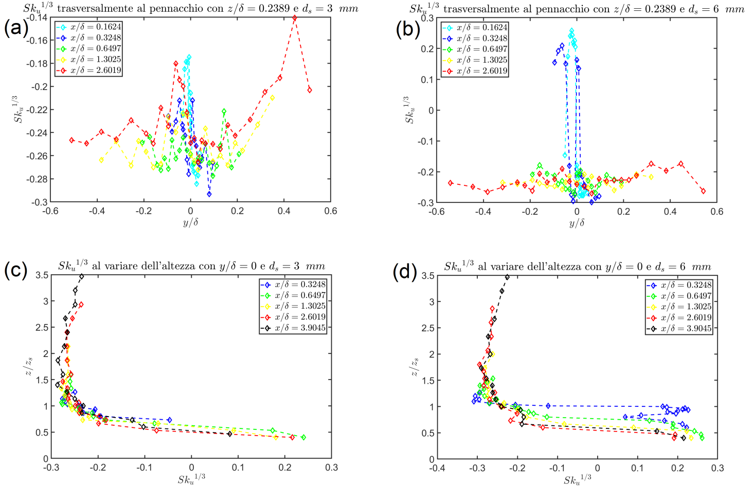
Figura 68: Grafici andamento Sk_u^{1/3} trasversalmente al pennacchio e al variare dell'altezza per d_s = 3 \text{ mm} e d_s = 6 \text{ mm} . In particolare: (a) Andamento di Sk_u^{1/3} per z/\delta = 0.2389 e d_s = 3 \text{ mm} , (b) Andamento di Sk_u^{1/3} per z/\delta = 0.2389 e d_s = 6 \text{ mm} , (c) Andamento di Sk_u^{1/3} per y/\delta = 0 e d_s = 3 \text{ mm} , (d) Andamento di Sk_u^{1/3} per y/\delta = 0 e d_s = 6 \text{ mm}
