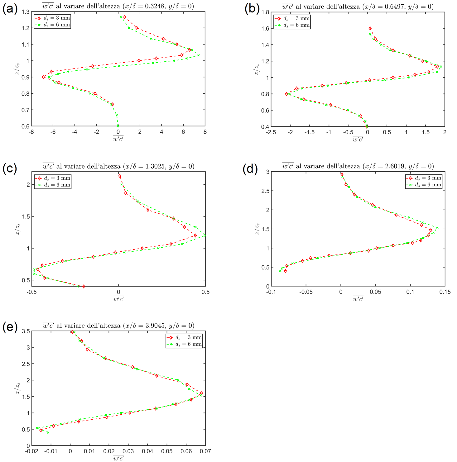
Figura 22: Grafici andamento \overline{w'c'} al variare dell'altezza per le cinque diverse sezioni per d_s = 3 mm e d_s = 6 mm, con y/\delta = 0 . In particolare: (a) Andamento di \overline{w'c'} per x/\delta = 0.3248 , (b) Andamento di \overline{w'c'} per x/\delta = 0.6497 , (c) Andamento di \overline{w'c'} per x/\delta = 1.3025 , (d) Andamento di \overline{w'c'} per x/\delta = 2.6019 , (e) Andamento di \overline{w'c'} per x/\delta = 3.9045
