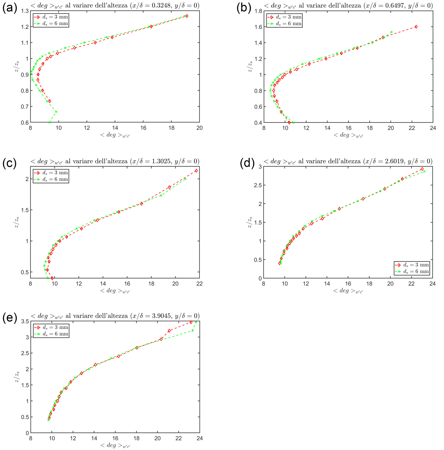
Figura 58: Grafici andamento \langle deg \rangle_{w'c'} al variare dell'altezza per le cinque diverse sezioni per d_s = 3 \text{ mm} e d_s = 6 \text{ mm} , con y/\delta = 0 . In particolare: (a) Andamento di \langle deg \rangle_{w'c'} per x/\delta = 0.3248 , (b) Andamento di \langle deg \rangle_{w'c'} per x/\delta = 0.6497 , (c) Andamento di \langle deg \rangle_{w'c'} per x/\delta = 1.3025 , (d) Andamento di \langle deg \rangle_{w'c'} per x/\delta = 2.6019 , (e) Andamento di \langle deg \rangle_{w'c'} per x/\delta = 3.9045
