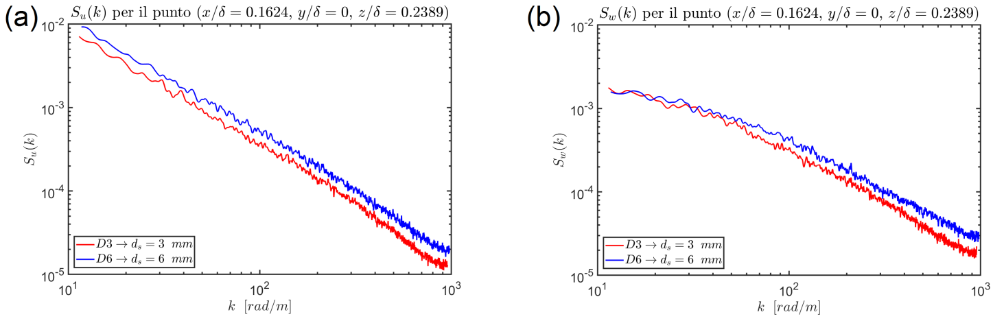
Figura 34: Grafici andamento S_u(k) e S_w(k) per d_s = 3 \text{ mm} e d_s = 6 \text{ mm} , per il punto (x/\delta = 0.1624, y/\delta = 0, z/\delta = 0.2389) . In particolare: (a) Andamento di S_u(k) , (b) Andamento di S_w(k)
