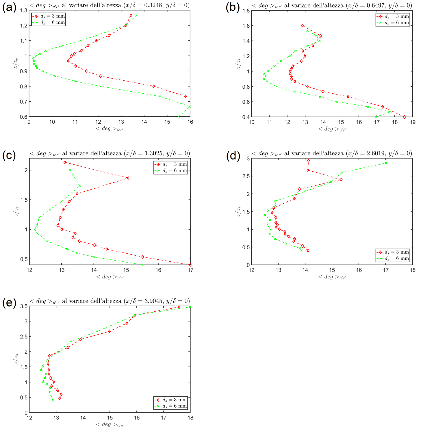
Figura 59: Grafici andamento \langle \deg \rangle_{u'c'} al variare dell'altezza per le cinque diverse sezioni per d_s = 3 \text{ mm} e d_s = 6 \text{ mm} , con y/\delta = 0 . In particolare: (a) Andamento di \langle \deg \rangle_{u'c'} per x/\delta = 0.3248 , (b) Andamento di \langle \deg \rangle_{u'c'} per x/\delta = 0.6497 , (c) Andamento di \langle \deg \rangle_{u'c'} per x/\delta = 1.3025 , (d) Andamento di \langle \deg \rangle_{u'c'} per x/\delta = 2.6019 , (e) Andamento di \langle \deg \rangle_{u'c'} per x/\delta = 3.9045
