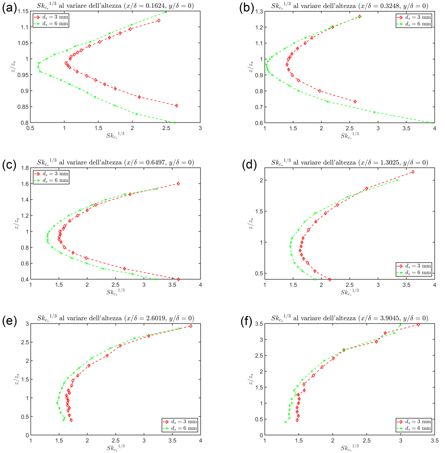
Figura 31: Grafici andamento Sk_{c*} al variare dell'altezza per le sei diverse sezioni per d_s = 3 \text{ mm} e d_s = 6 \text{ mm} , con y/\delta = 0 . In particolare: (a) Andamento di Sk_{c*} per x/\delta = 0.1624 , (b) Andamento di Sk_{c*} per x/\delta = 0.3248 , (c) Andamento di Sk_{c*} per x/\delta = 0.6497 , (d) Andamento di Sk_{c*} per x/\delta = 1.3025 , (e) Andamento di Sk_{c*} per x/\delta = 2.6019 , (f) Andamento di Sk_{c*} per x/\delta = 3.9045
