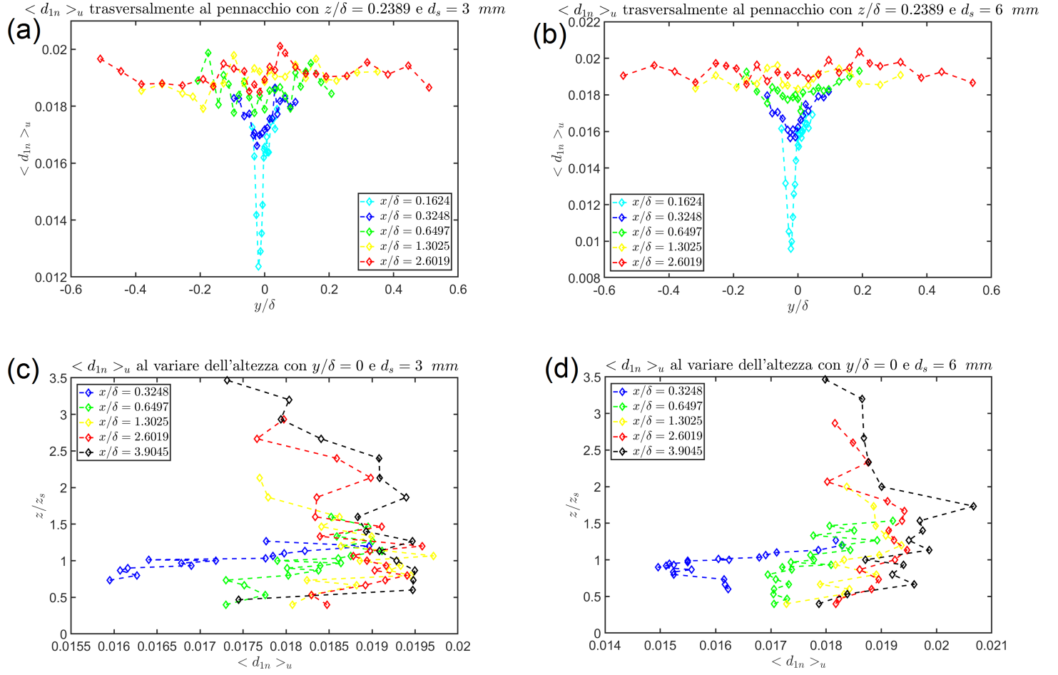
Figura 48: Grafici andamento \langle d_{1n} \rangle_u trasversalmente al pennacchio e al variare dell'altezza per d_s = 3 \text{ mm} e d_s = 6 \text{ mm} . In particolare: (a) Andamento di \langle d_{1n} \rangle_u per z/\delta = 0.2389 e d_s = 3 \text{ mm} , (b) Andamento di \langle d_{1n} \rangle_u per z/\delta = 0.2389 e d_s = 6 \text{ mm} , (c) Andamento di \langle d_{1n} \rangle_u per y/\delta = 0 e d_s = 3 \text{ mm} , (d) Andamento di \langle d_{1n} \rangle_u per y/\delta = 0 e d_s = 6 \text{ mm}
