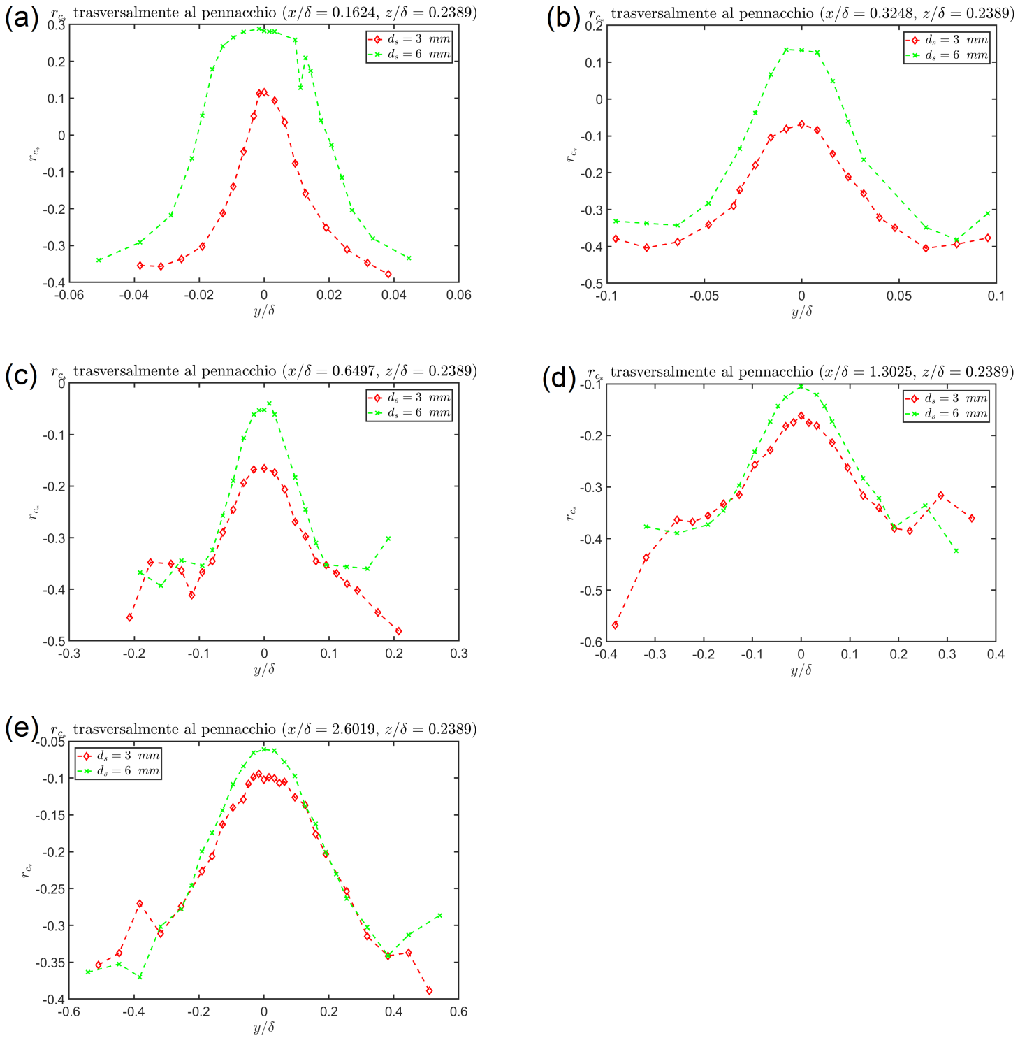
Figura 62: Grafici andamento r_{c*} trasversalmente al pennacchio per le cinque diverse sezioni per d_s = 3 \text{ mm} e d_s = 6 \text{ mm} , con z/\delta = 0.2389 ( z/z_s = 1 ). In particolare: (a) Andamento di r_{c*} per x/\delta = 0.1624 , (b) Andamento di r_{c*} per x/\delta = 0.3248 , (c) Andamento di r_{c*} per x/\delta = 0.6497 , (d) Andamento di r_{c*} per x/\delta = 1.3025 , (e) Andamento di r_{c*} per x/\delta = 2.6019
