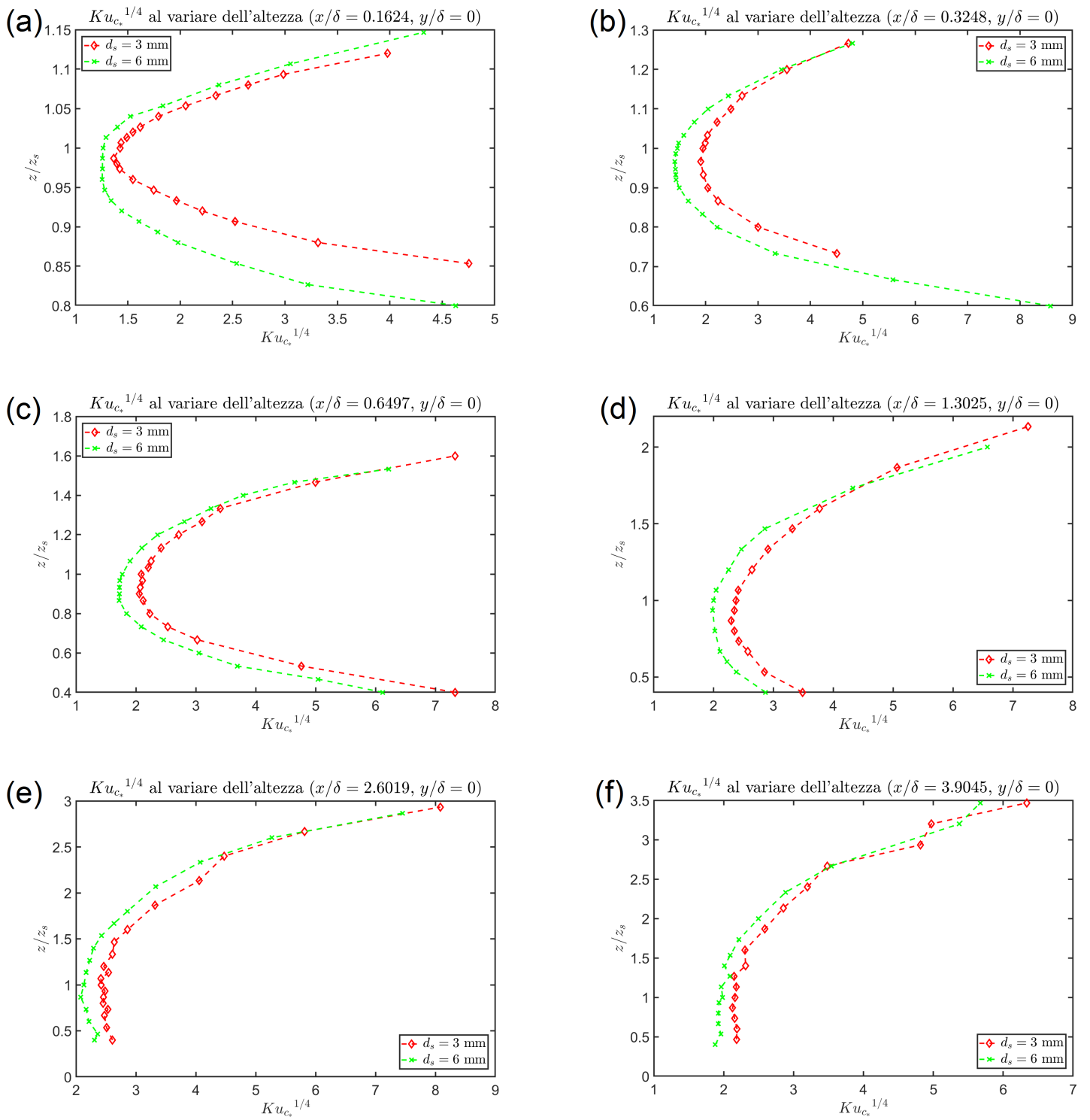
Figura 33: Grafici andamento Ku_{c_*}^{1/4} al variare dell'altezza per le sei diverse sezioni per d_s = 3 \text{ mm} e d_s = 6 \text{ mm} , con y/\delta = 0 . In particolare: (a) Andamento di Ku_{c_*}^{1/4} per x/\delta = 0.1624 , (b) Andamento di Ku_{c_*}^{1/4} per x/\delta = 0.3248 , (c) Andamento di Ku_{c_*}^{1/4} per x/\delta = 0.6497 , (d) Andamento di Ku_{c_*}^{1/4} per x/\delta = 1.3025 , (e) Andamento di Ku_{c_*}^{1/4} per x/\delta = 2.6019 , (f) Andamento di Ku_{c_*}^{1/4} per x/\delta = 3.9045
