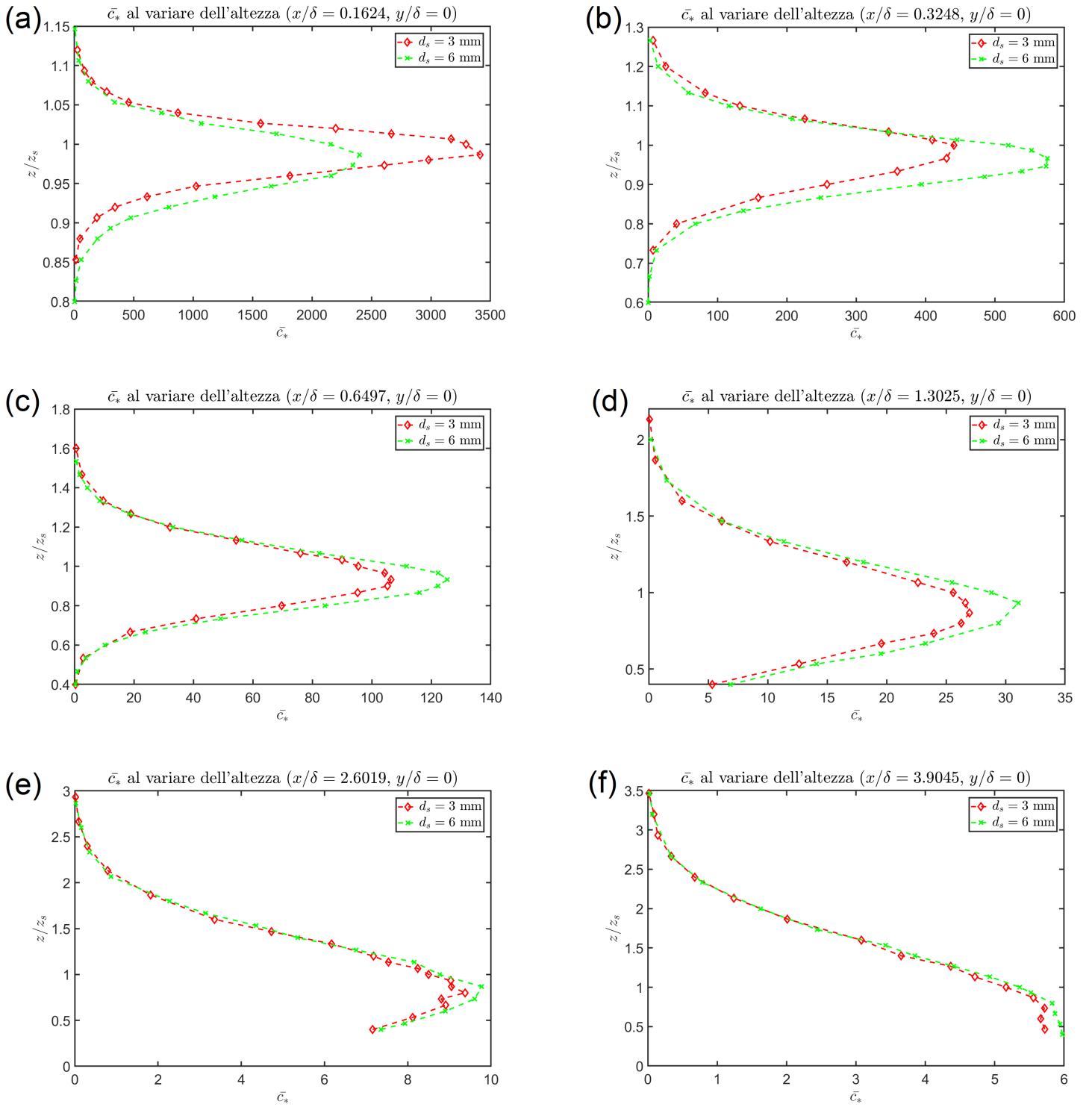
Figura 21: Grafici andamento \bar{c}_* al variare dell'altezza per le sei diverse sezioni per d_s = 3 \text{ mm} e d_s = 6 \text{ mm} , con y/\delta = 0 . In particolare: (a) Andamento di \bar{c}_* per x/\delta = 0.1624 , (b) Andamento di \bar{c}_* per x/\delta = 0.3248 , (c) Andamento di \bar{c}_* per x/\delta = 0.6497 , (d) Andamento di \bar{c}_* per x/\delta = 1.3025 , (e) Andamento di \bar{c}_* per x/\delta = 2.6019 , (f) Andamento di \bar{c}_* per x/\delta = 3.9045
