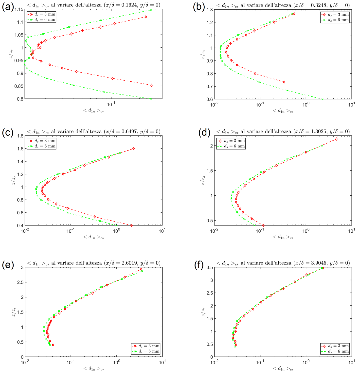
Figura 51: Grafici andamento \langle d_{1n} \rangle_{c^*} al variare dell'altezza per le sei diverse sezioni per d_s = 3 mm e d_s = 6 mm, con y/\delta = 0 . In particolare: (a) Andamento di \langle d_{1n} \rangle_{c^*} per x/\delta = 0.1624 , (b) Andamento di \langle d_{1n} \rangle_{c^*} per x/\delta = 0.3248 , (c) Andamento di \langle d_{1n} \rangle_{c^*} per x/\delta = 0.6497 , (d) Andamento di \langle d_{1n} \rangle_{c^*} per x/\delta = 1.3025 , (e) Andamento di \langle d_{1n} \rangle_{c^*} per x/\delta = 2.6019 , (f) Andamento di \langle d_{1n} \rangle_{c^*} per x/\delta = 3.9045
