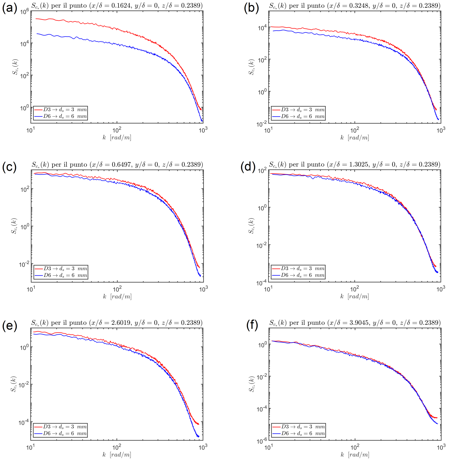
Figura 36: Grafici andamento S_{c_*}(k) per le sei diverse sezioni per d_s = 3 \text{ mm} e d_s = 6 \text{ mm} , con y/\delta = 0 e z/\delta = 0.2389 . In particolare: (a) Andamento di S_{c_*}(k) per x/\delta = 0.1624 , (b) Andamento di S_{c_*}(k) per x/\delta = 0.3248 , (c) Andamento di S_{c_*}(k) per x/\delta = 0.6497 , (d) Andamento di S_{c_*}(k) per x/\delta = 1.3025 , (e) Andamento di S_{c_*}(k) per x/\delta = 2.6019 , (f) Andamento di S_{c_*}(k) per x/\delta = 3.9045
