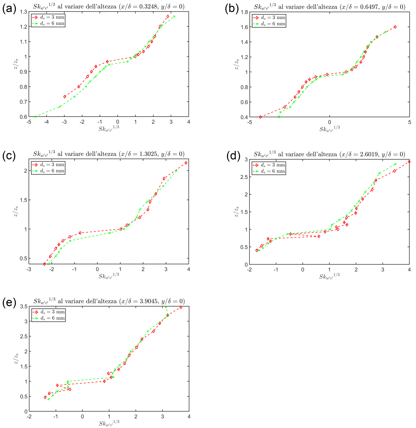
Figura 70: Grafici andamento Sk_{w'c'}^{1/3} al variare dell'altezza per le cinque diverse sezioni per d_s = 3 mm e d_s = 6 mm, con y/\delta = 0 . In particolare: (a) Andamento di Sk_{w'c'}^{1/3} per x/\delta = 0.3248 , (b) Andamento di Sk_{w'c'}^{1/3} per x/\delta = 0.6497 , (c) Andamento di Sk_{w'c'}^{1/3} per x/\delta = 1.3025 , (d) Andamento di Sk_{w'c'}^{1/3} per x/\delta = 2.6019 , (e) Andamento di Sk_{w'c'}^{1/3} per x/\delta = 3.9045
