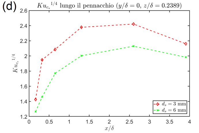
Figura 14: Grafici andamento \bar{c}_* , \sigma_{c_*} , Sk_{c_*}^{1/3} e Ku_{c_*}^{1/4} lungo il pennacchio, con y/\delta = 0 e z/\delta = 0.2389 ( z/z_s = 1 ). In particolare: (a) Andamento di \bar{c}_* in scala semi-logaritmica, (b) Andamento di \sigma_{c_*} in scala semi-logaritmica, (c) Andamento di Sk_{c_*}^{1/3} , (d) Andamento di Ku_{c_*}^{1/4}
