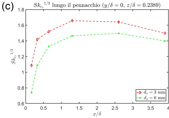
Figura 14: Grafici andamento \bar{c}_* , \sigma_{c_*} , Sk_{c_*}^{1/3} e Ku_{c_*}^{1/4} lungo il pennacchio, con y/\delta = 0 e z/\delta = 0.2389 ( z/z_s = 1 ). In particolare: (a) Andamento di \bar{c}_* in scala semi-logaritmica, (b) Andamento di \sigma_{c_*} in scala semi-logaritmica, (c) Andamento di Sk_{c_*}^{1/3} , (d) Andamento di Ku_{c_*}^{1/4}
