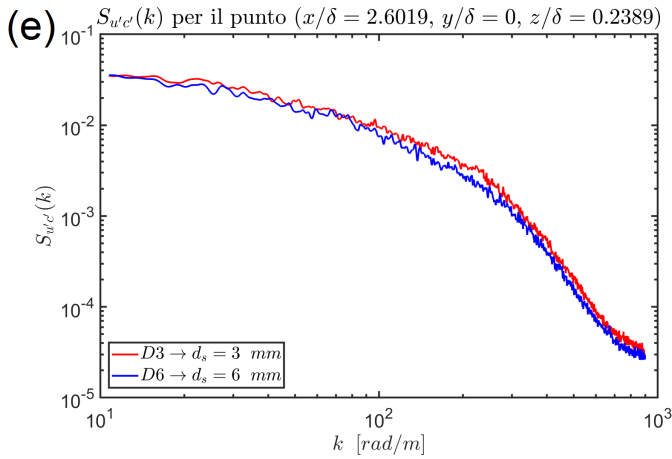
Figura 38: Grafici andamento S_{u'c'}(k) per le sei diverse sezioni per d_s = 3 \text{ mm} e d_s = 6 \text{ mm} , con y/\delta = 0 e z/\delta = 0.2389 . In particolare: (a) Andamento di S_{u'c'}(k) per x/\delta = 0.1624 , (b) Andamento di S_{u'c'}(k) per x/\delta = 0.3248 , (c) Andamento di S_{u'c'}(k) per x/\delta = 0.6497 , (d) Andamento di S_{u'c'}(k) per x/\delta = 1.3025 , (e) Andamento di S_{u'c'}(k) per x/\delta = 2.6019 , (f) Andamento di S_{u'c'}(k) per x/\delta = 3.9045
