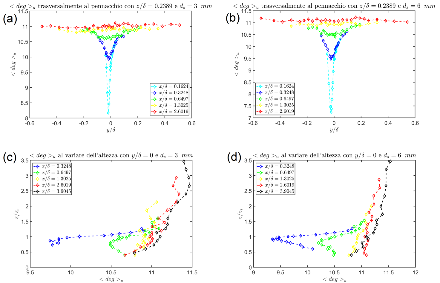
Figura 54: Grafici andamento \langle deg \rangle_u trasversalmente al pennacchio e al variare dell'altezza per d_s = 3 \text{ mm} e d_s = 6 \text{ mm} . In particolare: (a) Andamento di \langle deg \rangle_u per z/\delta = 0.2389 e d_s = 3 \text{ mm} , (b) Andamento di \langle deg \rangle_u per z/\delta = 0.2389 e d_s = 6 \text{ mm} , (c) Andamento di \langle deg \rangle_u per y/\delta = 0 e d_s = 3 \text{ mm} , (d) Andamento di \langle deg \rangle_u per y/\delta = 0 e d_s = 6 \text{ mm}
