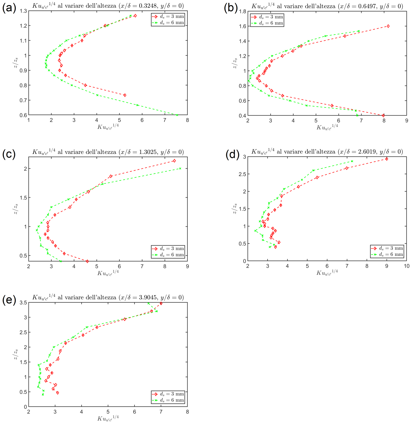
Figura 75: Grafici andamento K u_{w'c'}^{1/4} al variare dell'altezza per le cinque diverse sezioni per d_s = 3 mm e d_s = 6 mm, con y/\delta = 0 . In particolare: (a) Andamento di K u_{w'c'}^{1/4} per x/\delta = 0.3248 , (b) Andamento di K u_{w'c'}^{1/4} per x/\delta = 0.6497 , (c) Andamento di K u_{w'c'}^{1/4} per x/\delta = 1.3025 , (d) Andamento di K u_{w'c'}^{1/4} per x/\delta = 2.6019 , (e) Andamento di K u_{w'c'}^{1/4} per x/\delta = 3.9045
