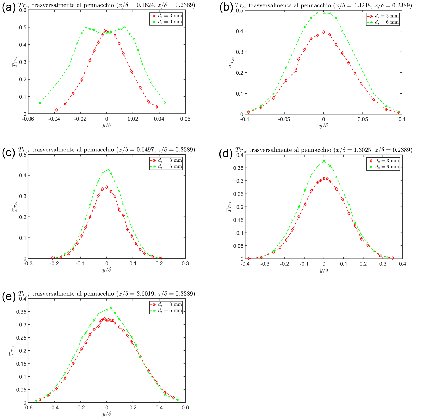
Figura 44: Grafici andamento Tr_{c*} trasversalmente al pennacchio per le cinque diverse sezioni per d_s = 3 \text{ mm} e d_s = 6 \text{ mm} , con z/\delta = 0.2389 ( z/z_s = 1 ). In particolare: (a) Andamento di Tr_{c*} per x/\delta = 0.1624 , (b) Andamento di Tr_{c*} per x/\delta = 0.3248 , (c) Andamento di Tr_{c*} per x/\delta = 0.6497 , (d) Andamento di Tr_{c*} per x/\delta = 1.3025 , (e) Andamento di Tr_{c*} per x/\delta = 2.6019
