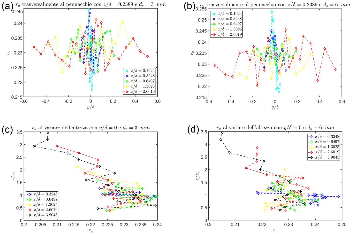
Figura 60: Grafici andamento r_u trasversalmente al pennacchio e al variare dell'altezza per d_s = 3 \text{ mm} e d_s = 6 \text{ mm} . In particolare: (a) Andamento di r_u per z/\delta = 0.2389 e d_s = 3 \text{ mm} , (b) Andamento di r_u per z/\delta = 0.2389 e d_s = 6 \text{ mm} , (c) Andamento di r_u per y/\delta = 0 e d_s = 3 \text{ mm} , (d) Andamento di r_u per y/\delta = 0 e d_s = 6 \text{ mm}
