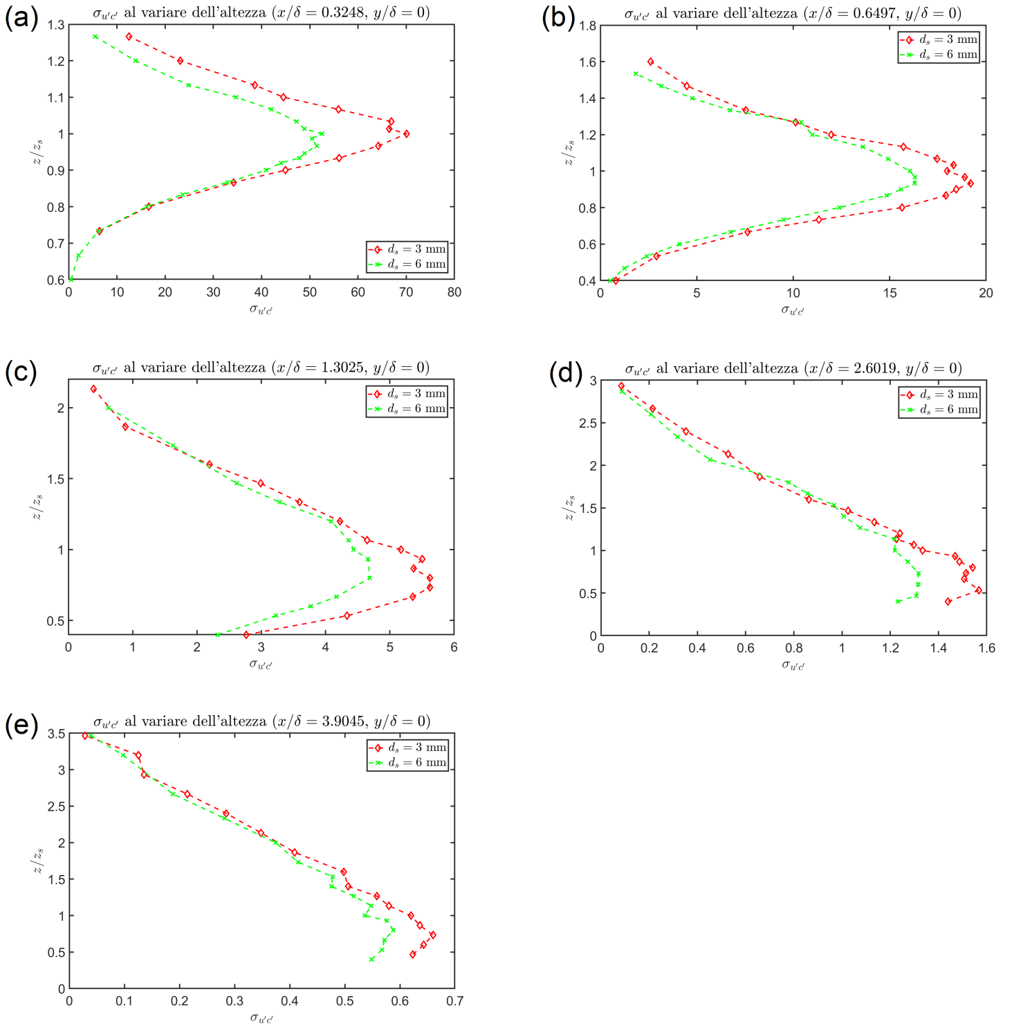
Figura 29: Grafici andamento \sigma_{u'c'} al variare dell'altezza per le cinque diverse sezioni per d_s = 3 \text{ mm} e d_s = 6 \text{ mm} , con y/\delta = 0 . In particolare: (a) Andamento di \sigma_{u'c'} per x/\delta = 0.3248 , (b) Andamento di \sigma_{u'c'} per x/\delta = 0.6497 , (c) Andamento di \sigma_{u'c'} per x/\delta = 1.3025 , (d) Andamento di \sigma_{u'c'} per x/\delta = 2.6019 , (e) Andamento di \sigma_{u'c'} per x/\delta = 3.9045
