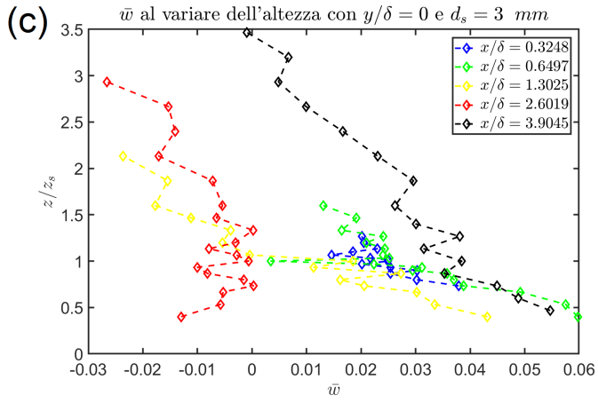
Figura 19: Grafici andamento \bar{w} trasversalmente al pennacchio e al variare dell'altezza per d_s = 3 \text{ mm} e d_s = 6 \text{ mm} . In particolare: (a) Andamento di \bar{w} per z/\delta = 0.2389 e d_s = 3 \text{ mm} , (b) Andamento di \bar{w} per z/\delta = 0.2389 e d_s = 6 \text{ mm} , (c) Andamento di \bar{w} per y/\delta = 0 e d_s = 3 \text{ mm} , (d) Andamento di \bar{w} per y/\delta = 0 e d_s = 6 \text{ mm}
