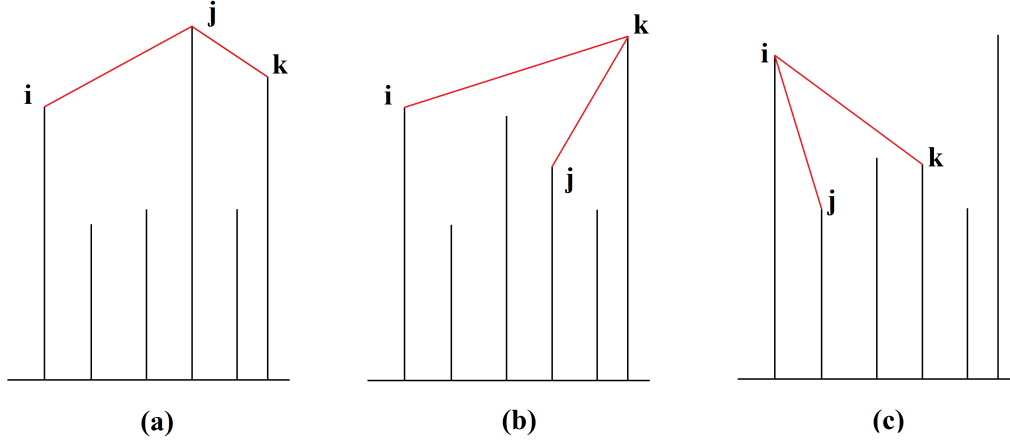
Figura 11: Rappresentazione delle tre tipologie di triple connesse, che non sono contemporaneamente triangoli. In particolare: (a) Il nodo i e il nodo k sono collegati indirettamente dal nodo j , (b) Il nodo i e il nodo j sono collegati indirettamente dal nodo k , (c) Il nodo j e il nodo k sono collegati indirettamente dal nodo i
