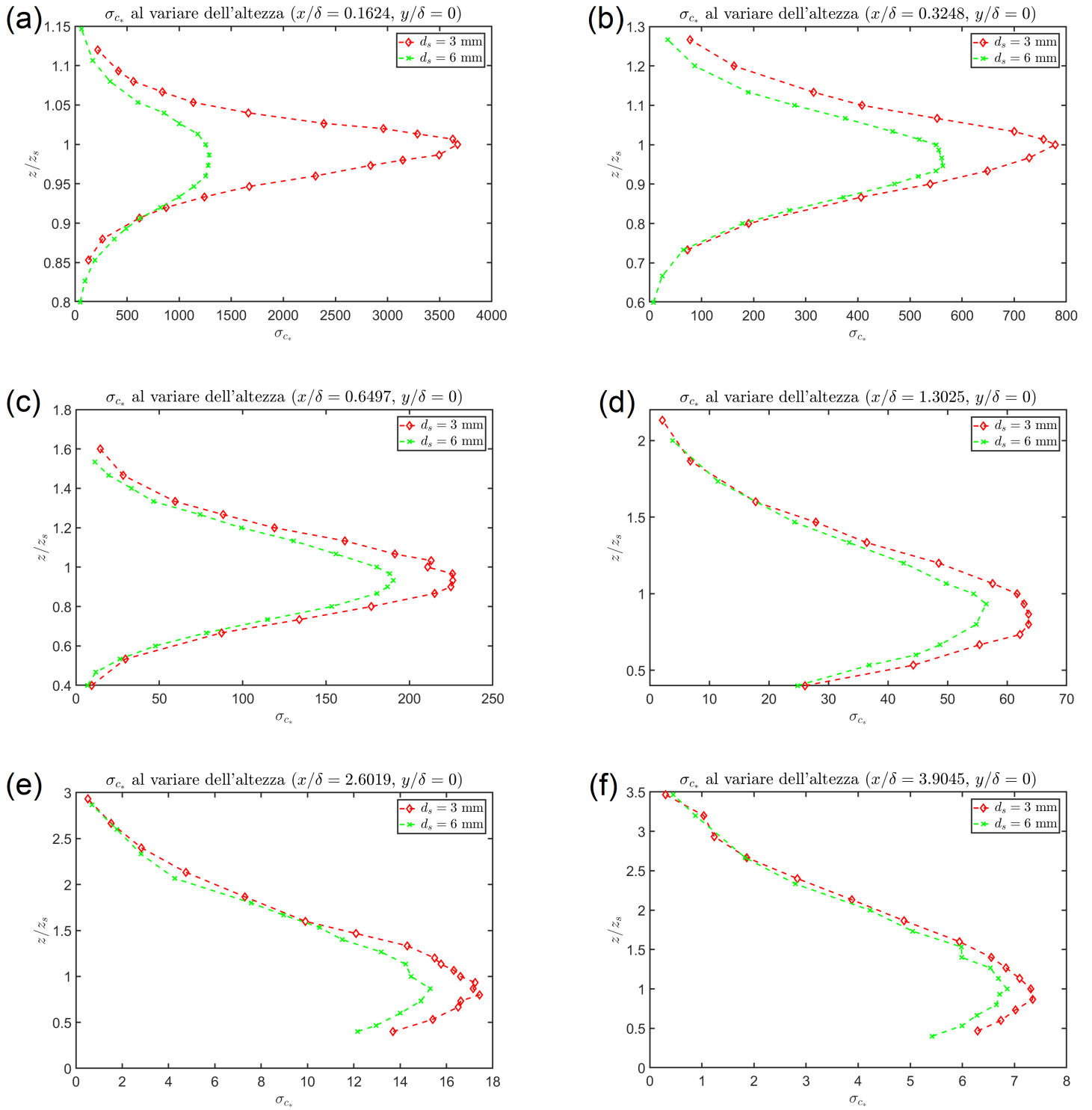
Figura 27: Grafici andamento \sigma_{c*} al variare dell'altezza per le sei diverse sezioni per d_s = 3 \text{ mm} e d_s = 6 \text{ mm} , con y/\delta = 0 . In particolare: (a) Andamento di \sigma_{c*} per x/\delta = 0.1624 , (b) Andamento di \sigma_{c*} per x/\delta = 0.3248 , (c) Andamento di \sigma_{c*} per x/\delta = 0.6497 , (d) Andamento di \sigma_{c*} per x/\delta = 1.3025 , (e) Andamento di \sigma_{c*} per x/\delta = 2.6019 , (f) Andamento di \sigma_{c*} per x/\delta = 3.9045
