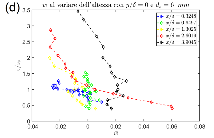
Figura 19: Grafici andamento \bar{w} trasversalmente al pennacchio e al variare dell'altezza per d_s = 3 \text{ mm} e d_s = 6 \text{ mm} . In particolare: (a) Andamento di \bar{w} per z/\delta = 0.2389 e d_s = 3 \text{ mm} , (b) Andamento di \bar{w} per z/\delta = 0.2389 e d_s = 6 \text{ mm} , (c) Andamento di \bar{w} per y/\delta = 0 e d_s = 3 \text{ mm} , (d) Andamento di \bar{w} per y/\delta = 0 e d_s = 6 \text{ mm}
