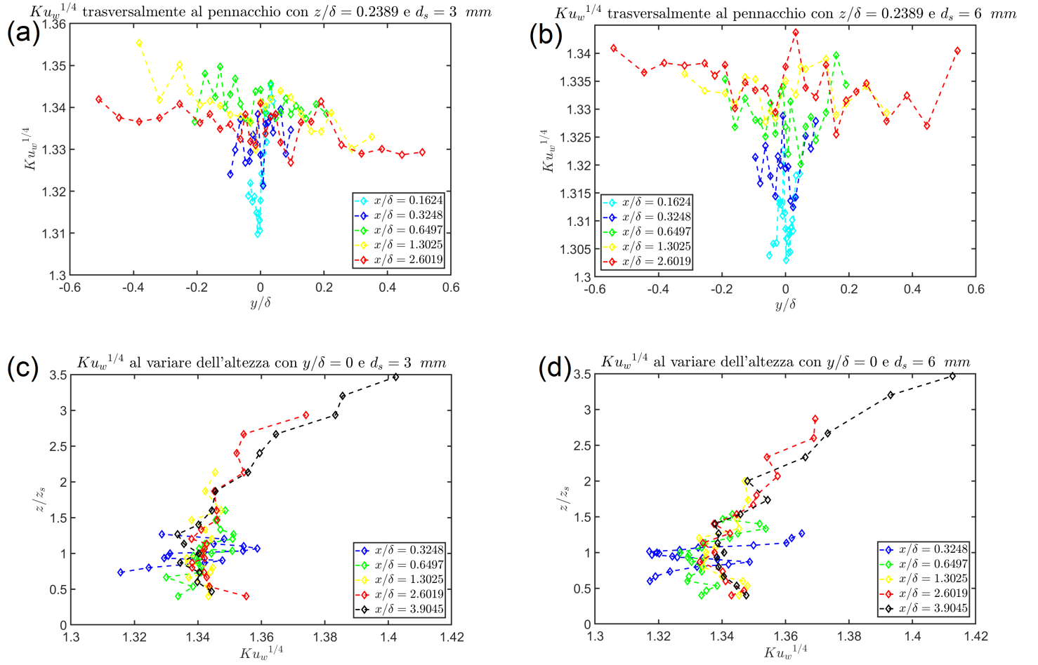
Figura 73: Grafici andamento Ku_w^{1/4} trasversalmente al pennacchio e al variare dell'altezza per d_s = 3 \text{ mm} e d_s = 6 \text{ mm} . In particolare: (a) Andamento di Ku_w^{1/4} per z/\delta = 0.2389 e d_s = 3 \text{ mm} , (b) Andamento di Ku_w^{1/4} per z/\delta = 0.2389 e d_s = 6 \text{ mm} , (c) Andamento di Ku_w^{1/4} per y/\delta = 0 e d_s = 3 \text{ mm} , (d) Andamento di Ku_w^{1/4} per y/\delta = 0 e d_s = 6 \text{ mm}
