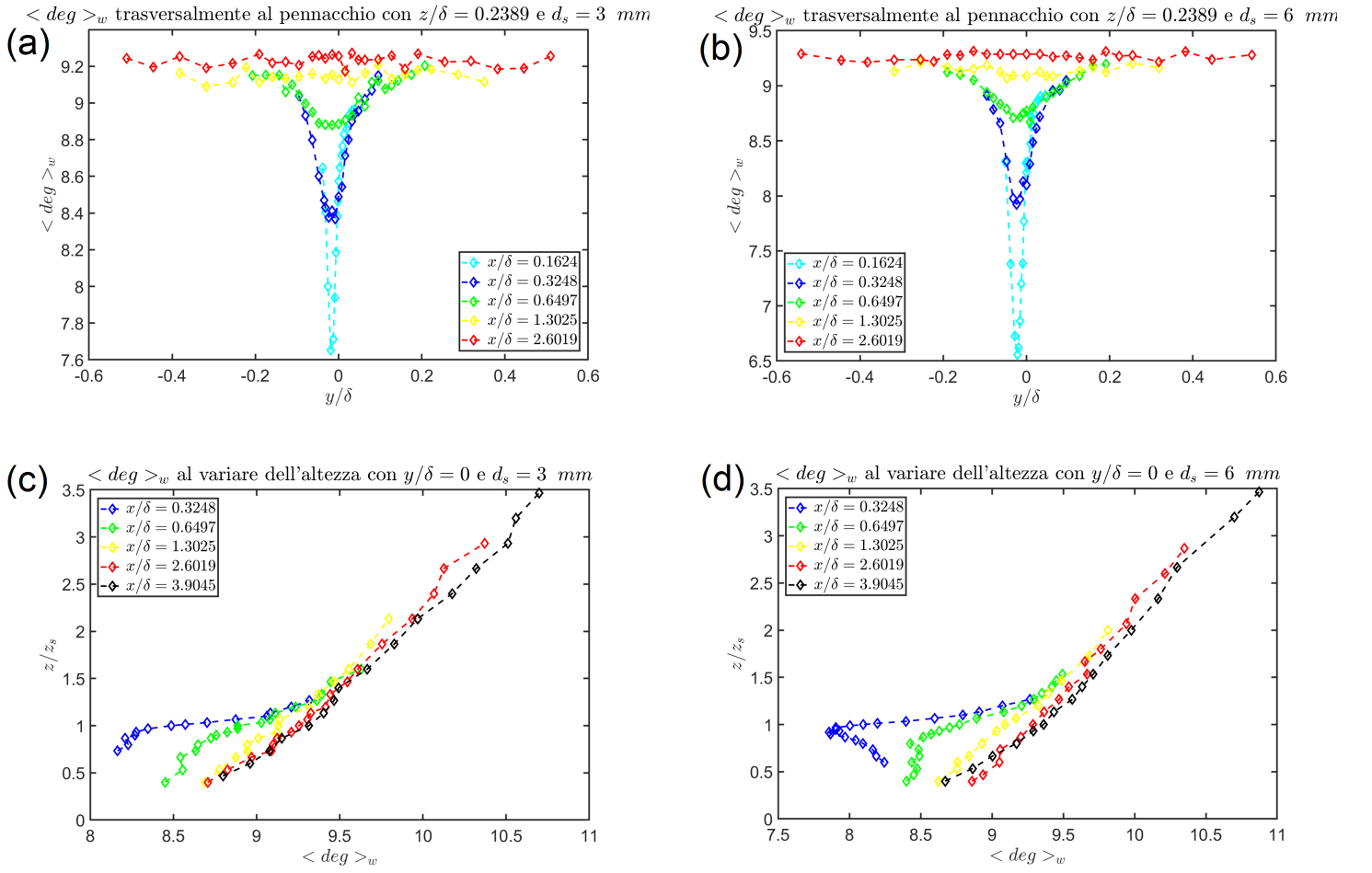
Figura 55: Grafici andamento \langle deg \rangle_w trasversalmente al pennacchio e al variare dell'altezza per d_s = 3 \text{ mm} e d_s = 6 \text{ mm} . In particolare: (a) Andamento di \langle deg \rangle_w per z/\delta = 0.2389 e d_s = 3 \text{ mm} , (b) Andamento di \langle deg \rangle_w per z/\delta = 0.2389 e d_s = 6 \text{ mm} , (c) Andamento di \langle deg \rangle_w per y/\delta = 0 e d_s = 3 \text{ mm} , (d) Andamento di \langle deg \rangle_w per y/\delta = 0 e d_s = 6 \text{ mm}
