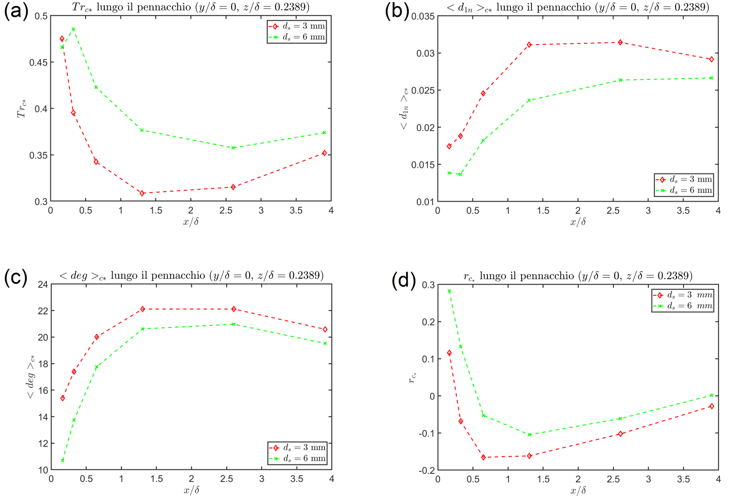
Figura 39: Grafici andamento Tr_{c*} , \langle d_{1n} \rangle_{c*} , \langle deg \rangle_{c*} e r_{c*} lungo il pennacchio, con y/\delta = 0 e z/\delta = 0.2389 ( z/z_s = 1 ). In particolare: (a) Andamento di Tr_{c*} , (b) Andamento di \langle d_{1n} \rangle_{c*} , (c) Andamento di \langle deg \rangle_{c*} , (d) Andamento di r_{c*} .
